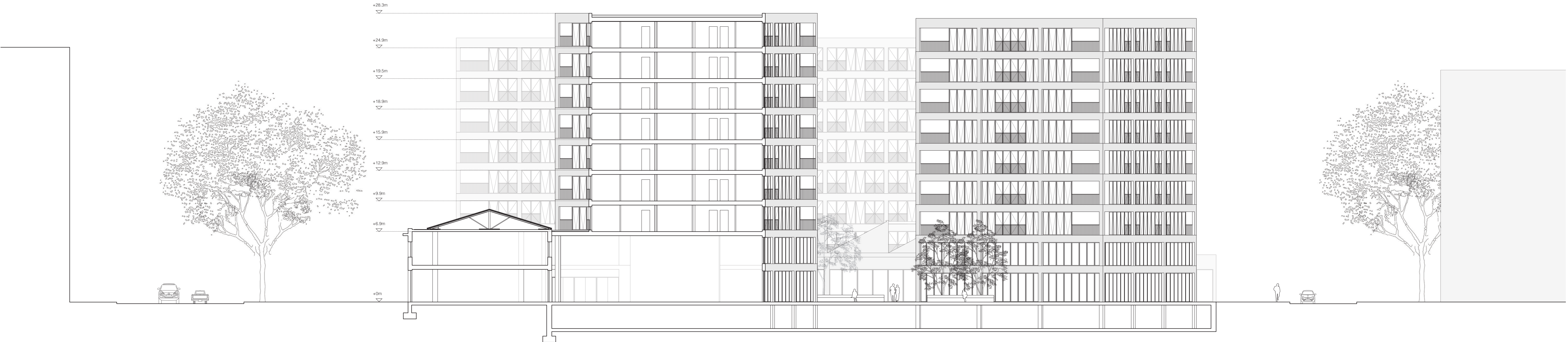
FabLab et ateliers éducatifs AA' 1:200
