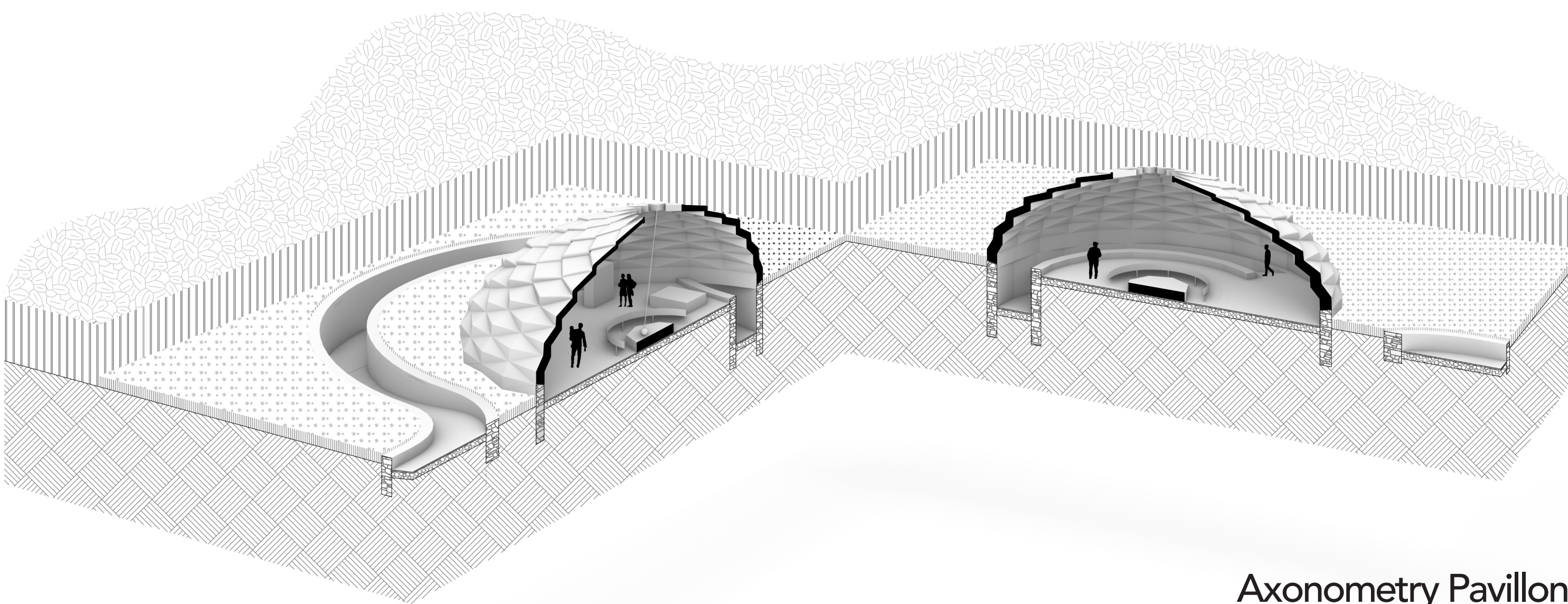
Axonometry Pavillon
