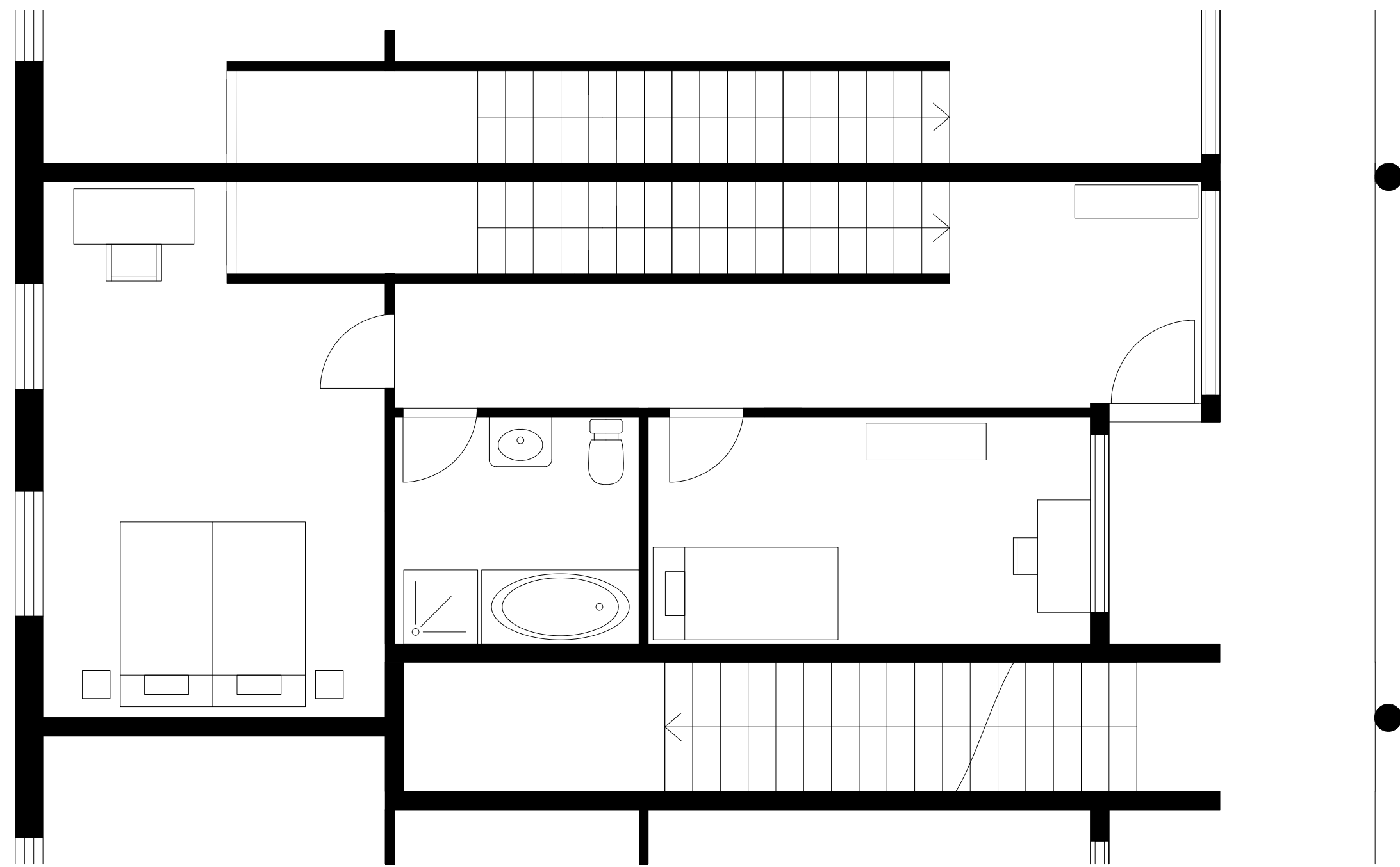
Typologie appartement duplex 120m² 1 : 50
