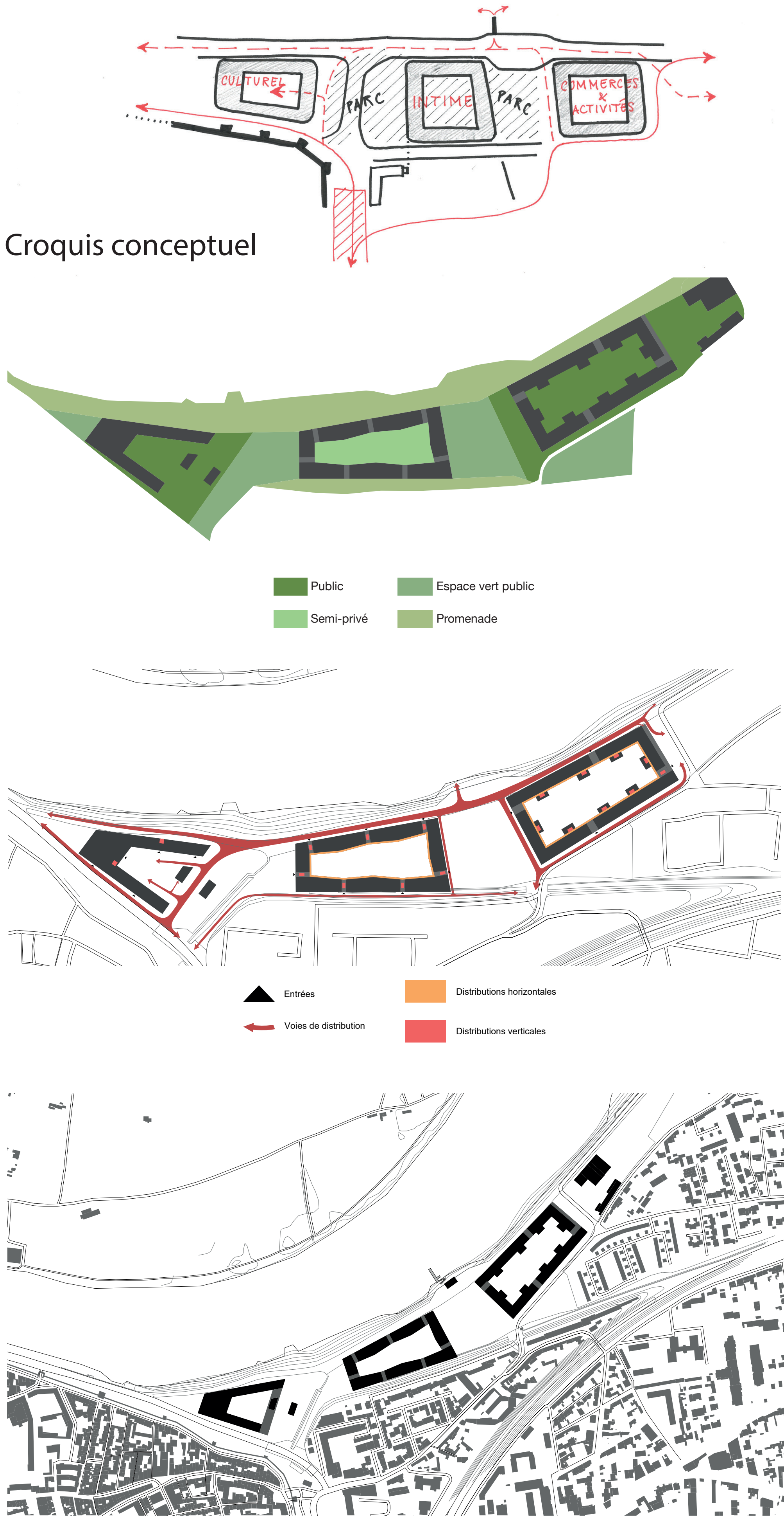
Plan de masse 1:5000
