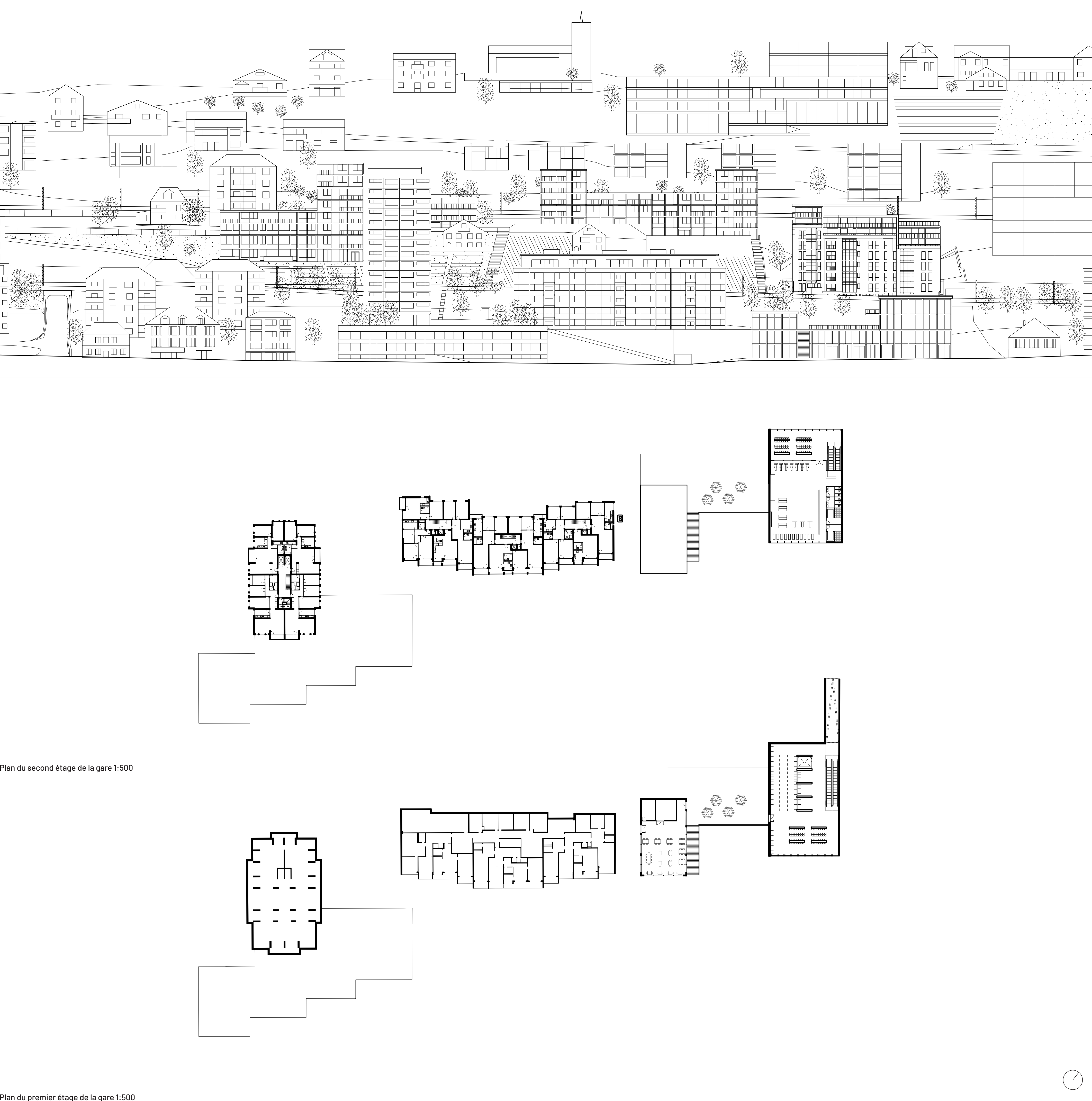
Plan du premier étage de la gare 1:500
