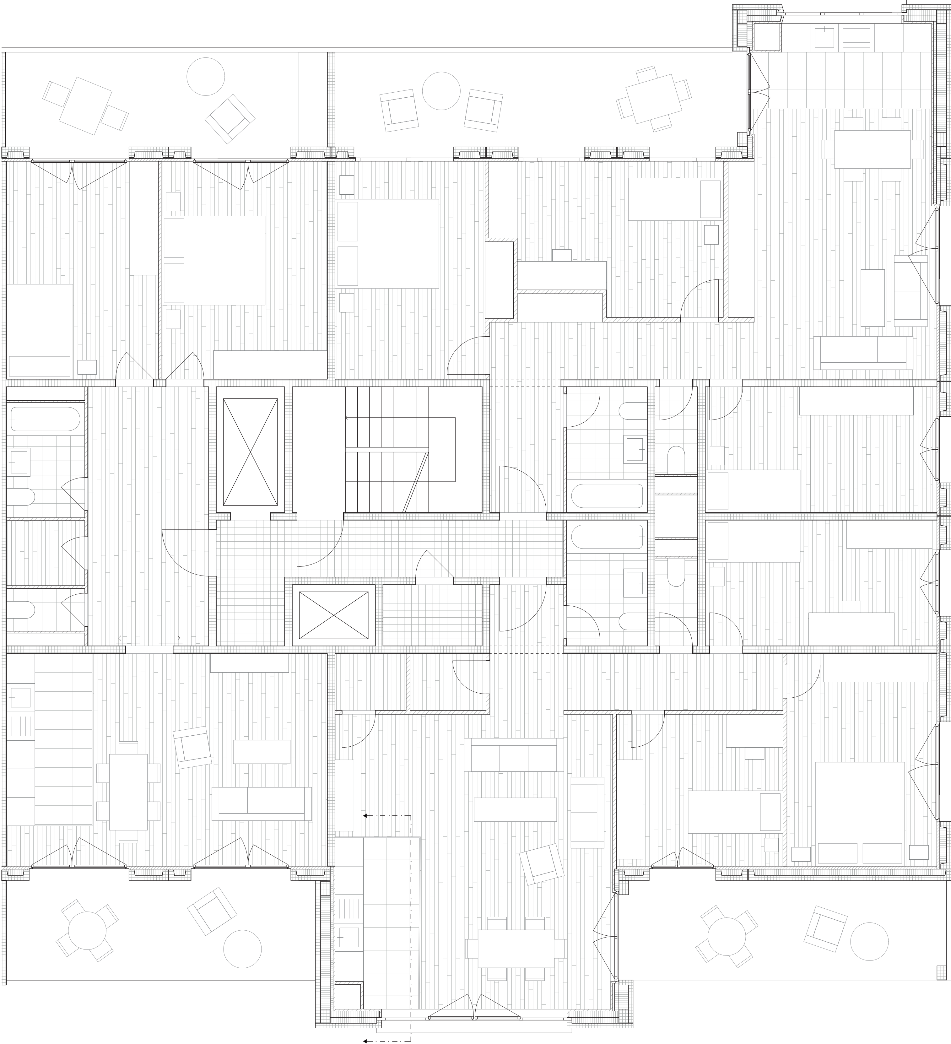
Plan d'appartements après rénovation 1:50
