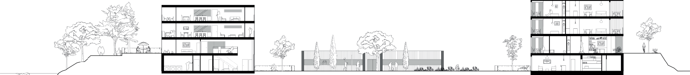
COUPE A 1:100
