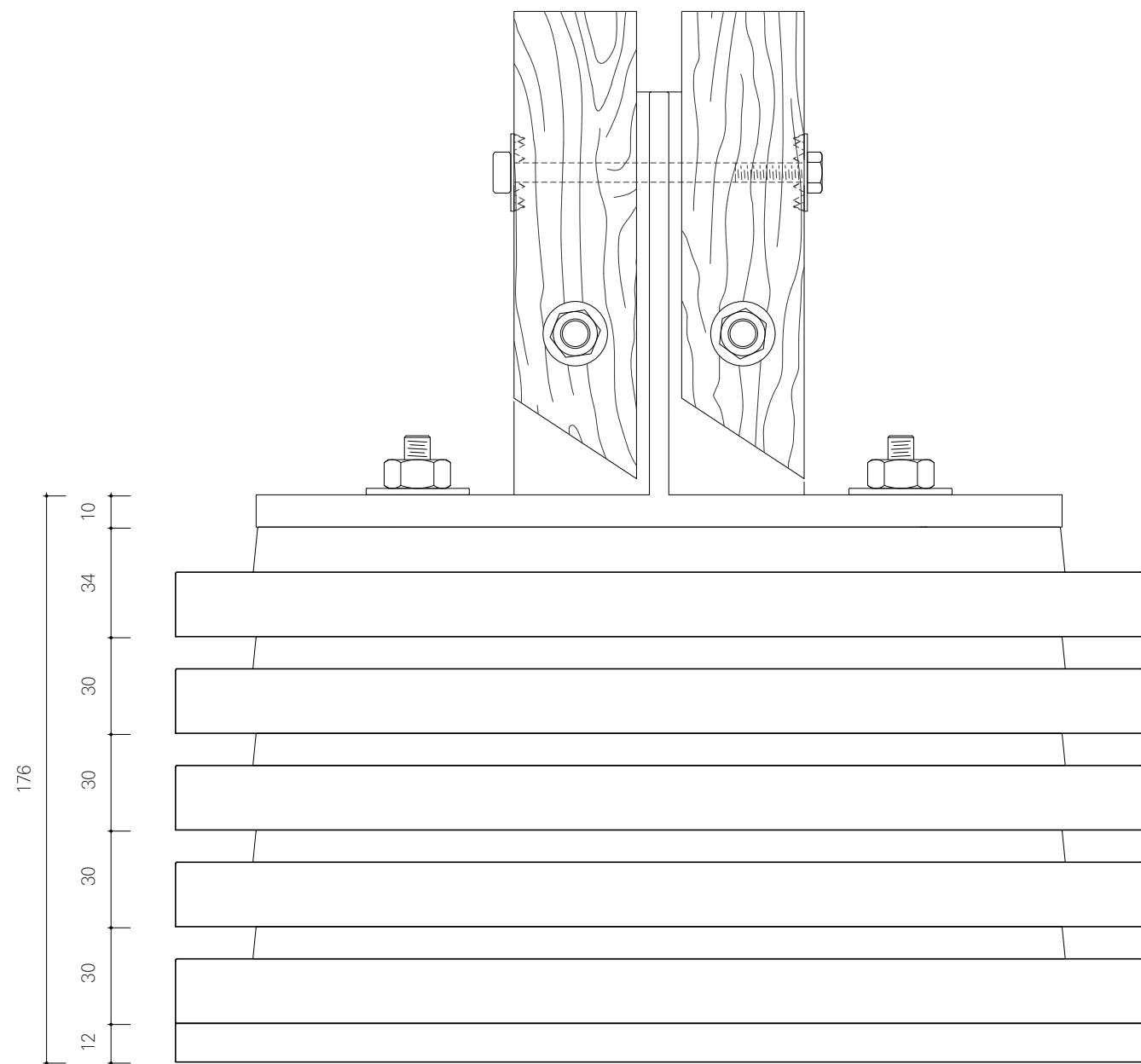
Elevation Ancre
