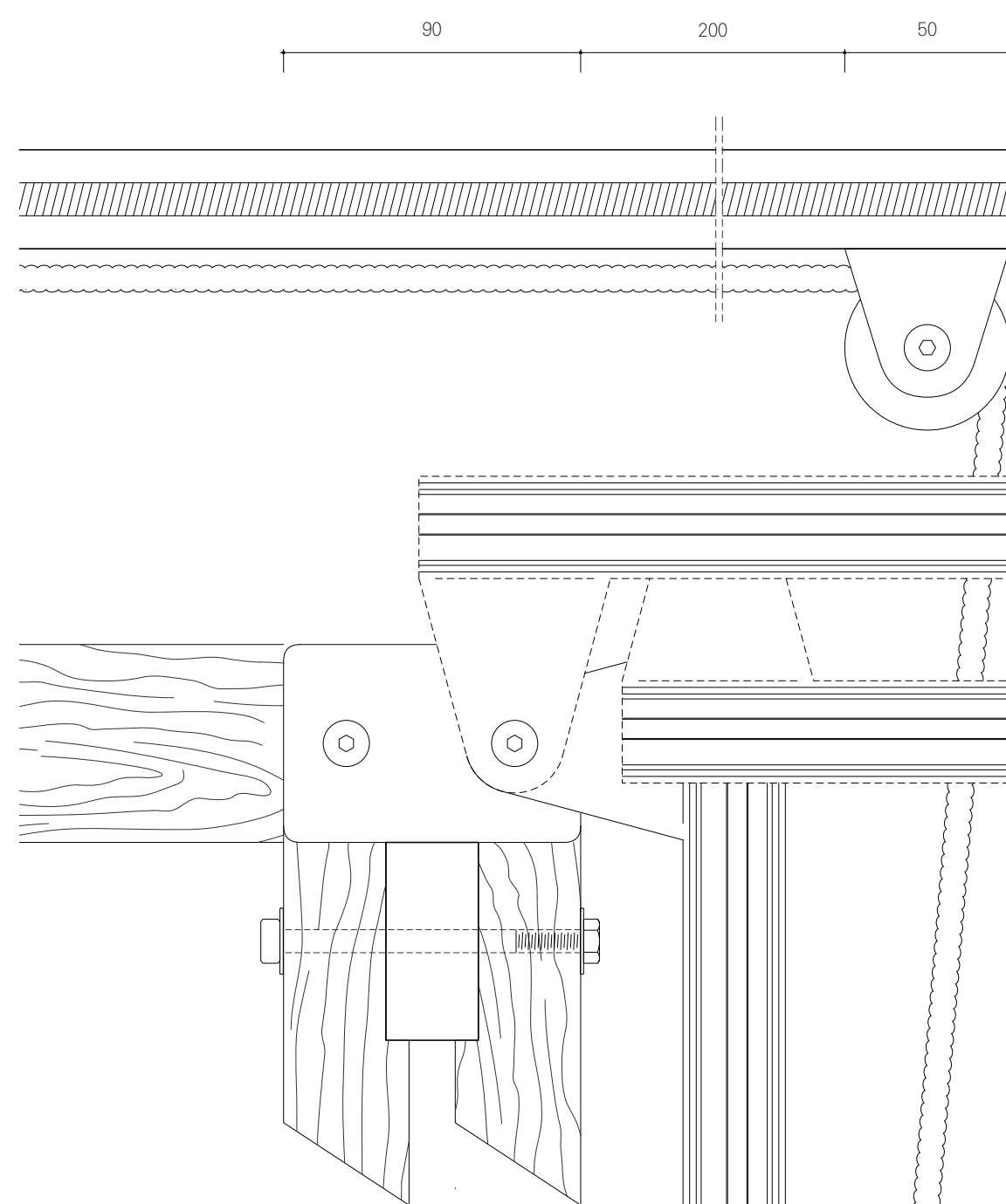
Coupe Façade
