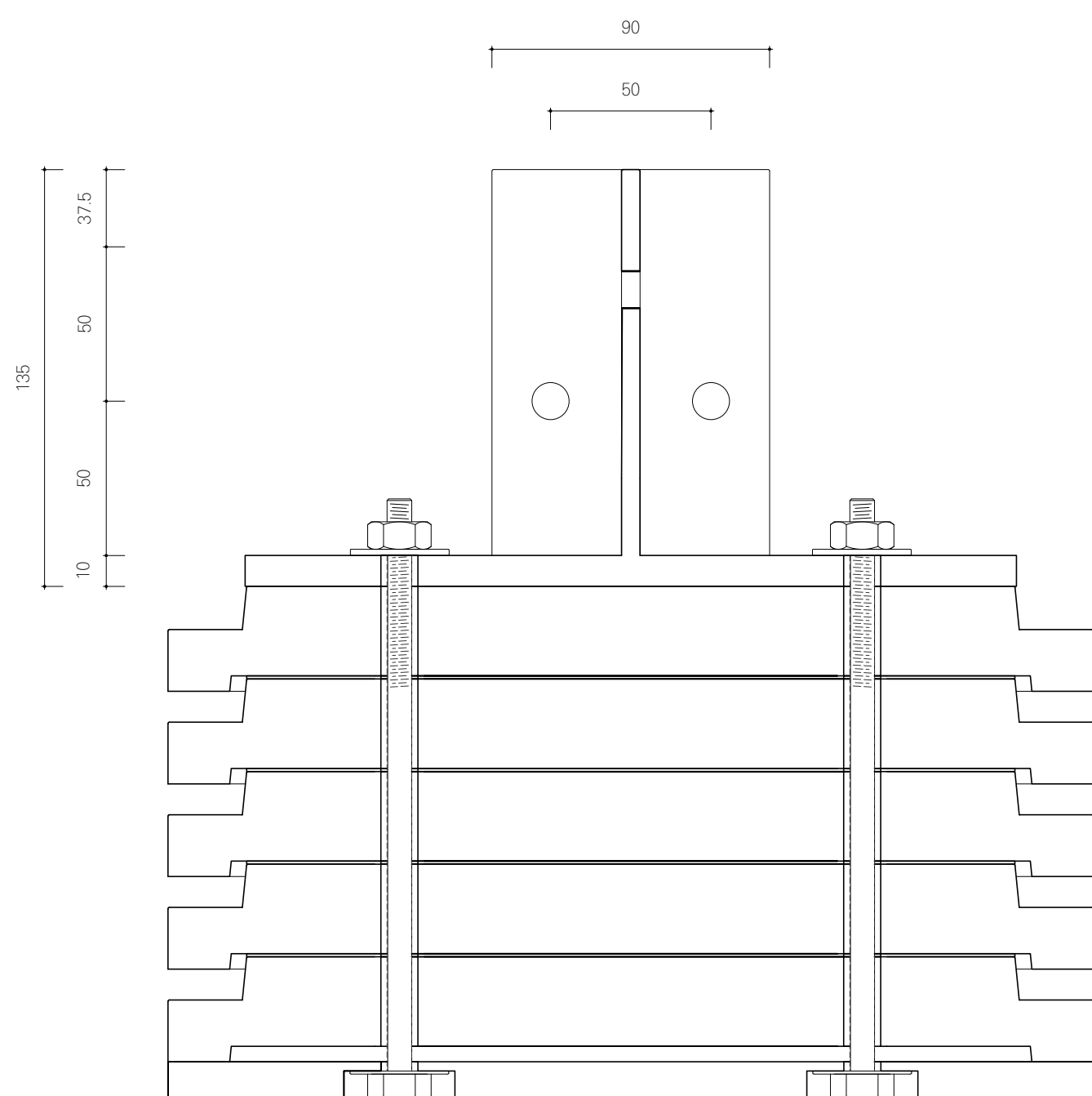
Coupe Ancre
