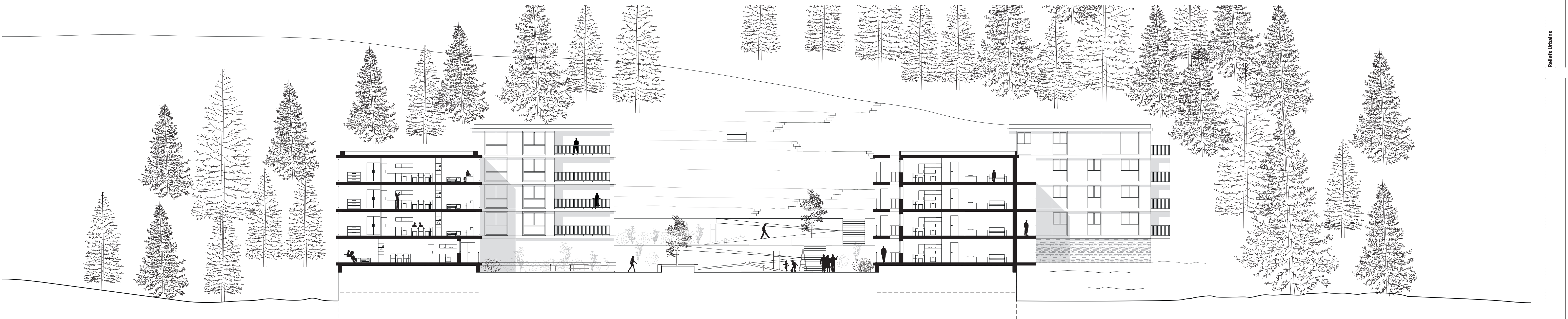
Coupe niveau 3 1:200
