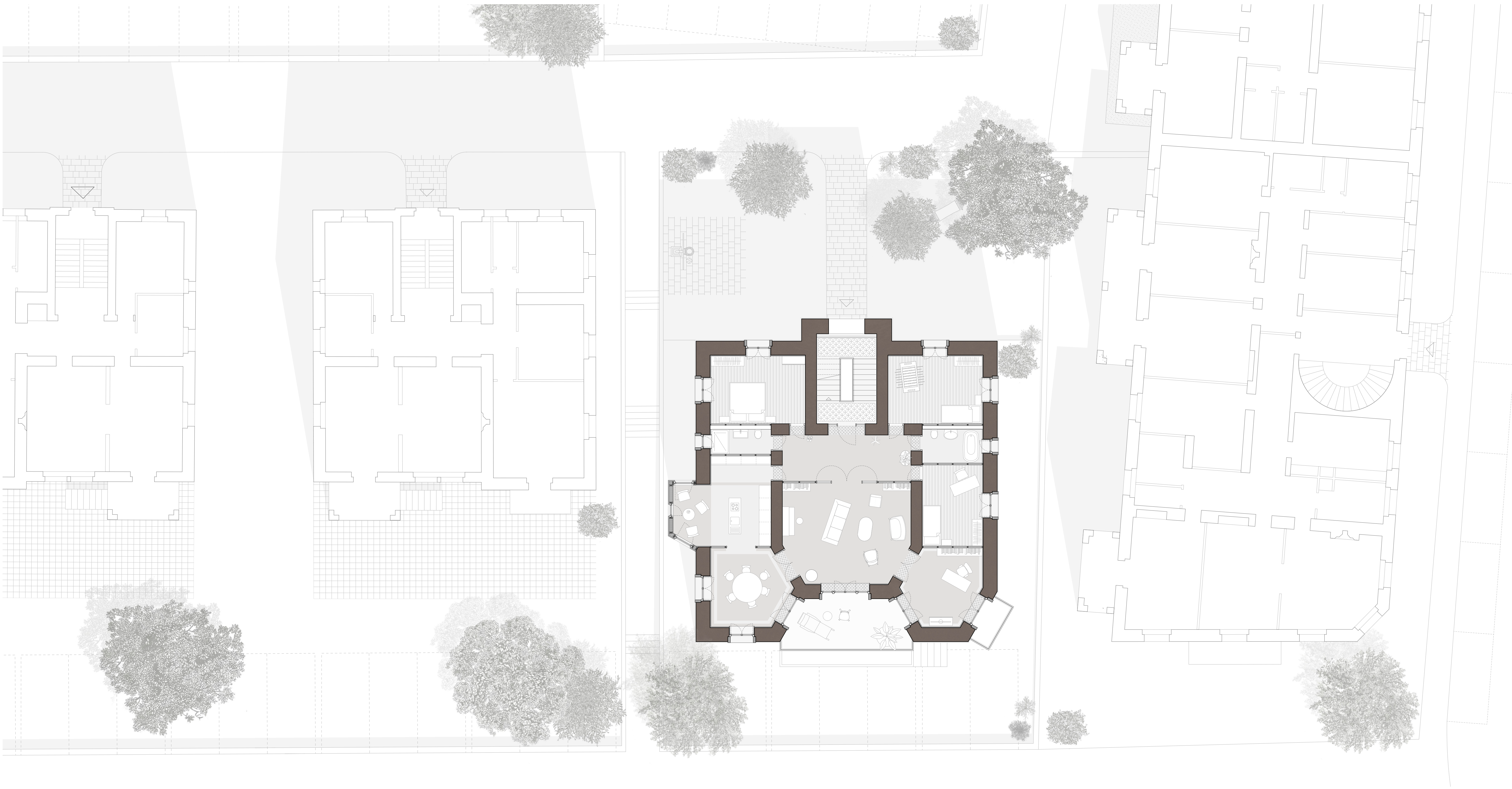
Plan du 2 ème étage - 1:100
