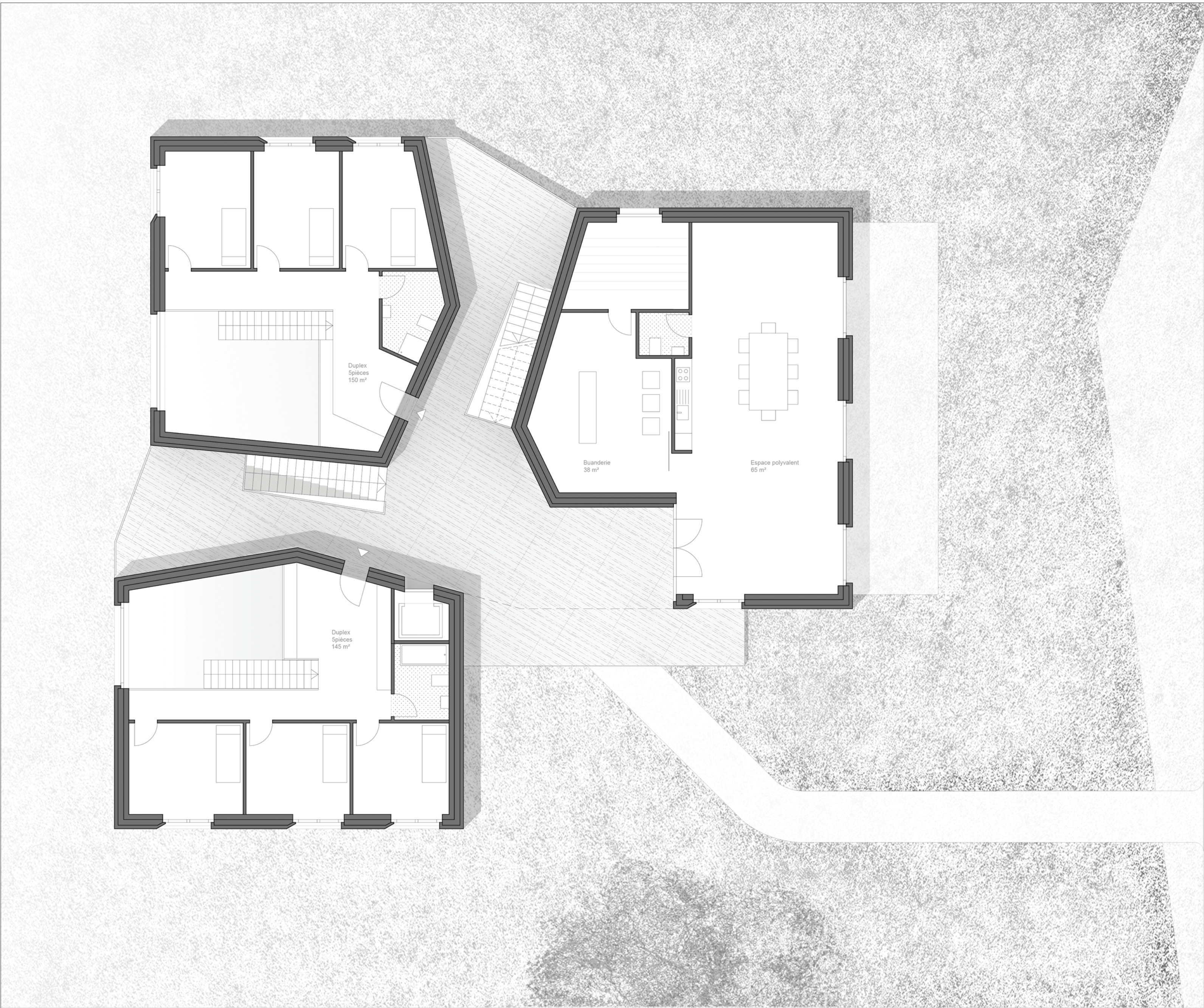
Plan du rez supérieur 1:100
