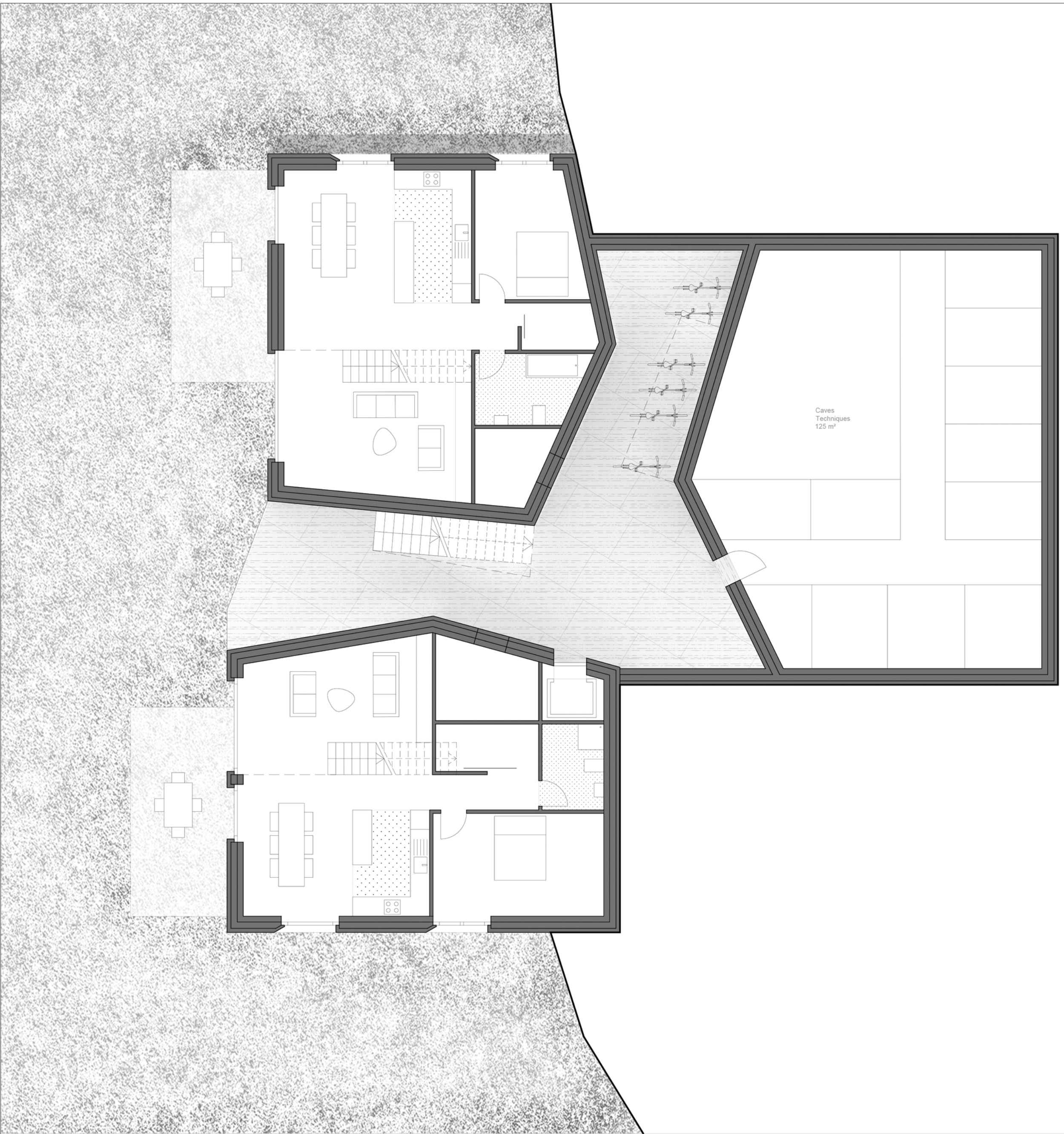
Plan du rez inférieur 1:100
