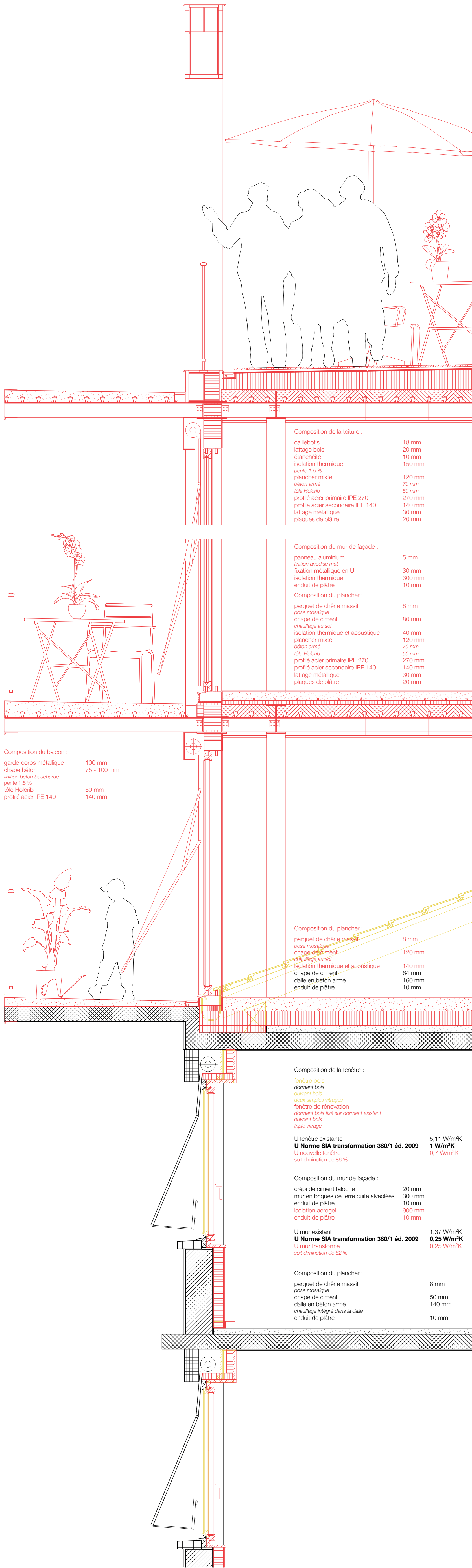
Coupe constructive rue de la Servette 1:20
