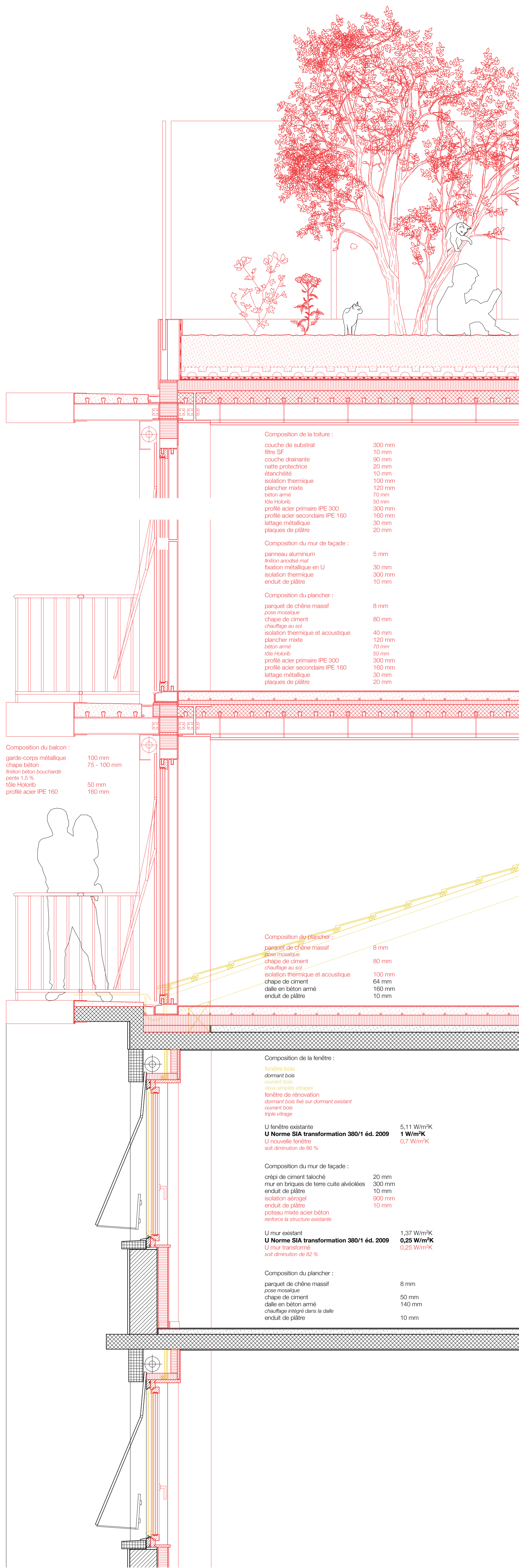
Coupe constructive rue Antoine-Carteret 1:20
