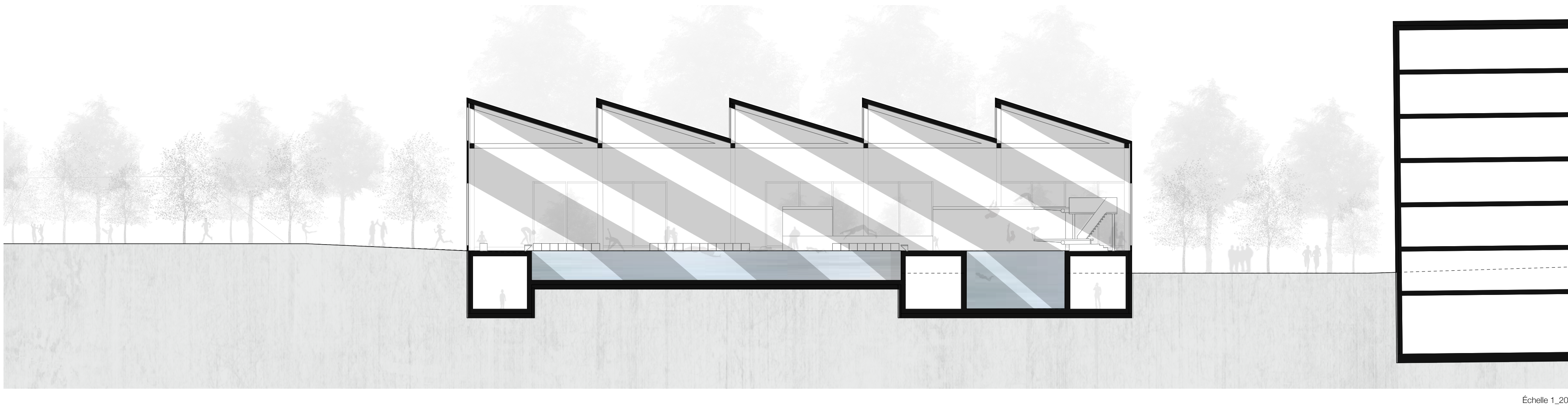
Coupe longitudinale CC
