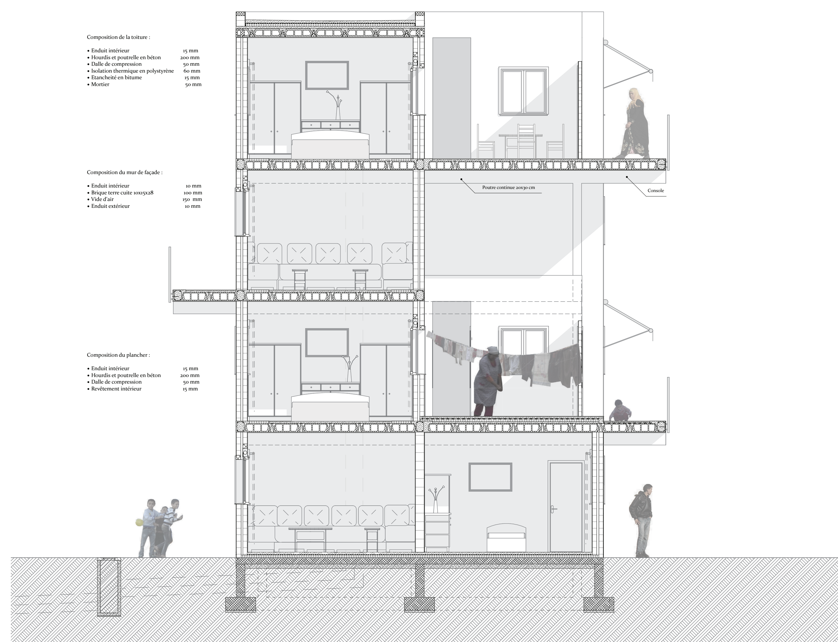
COUPE CONSTRUCTIVE 1:50
