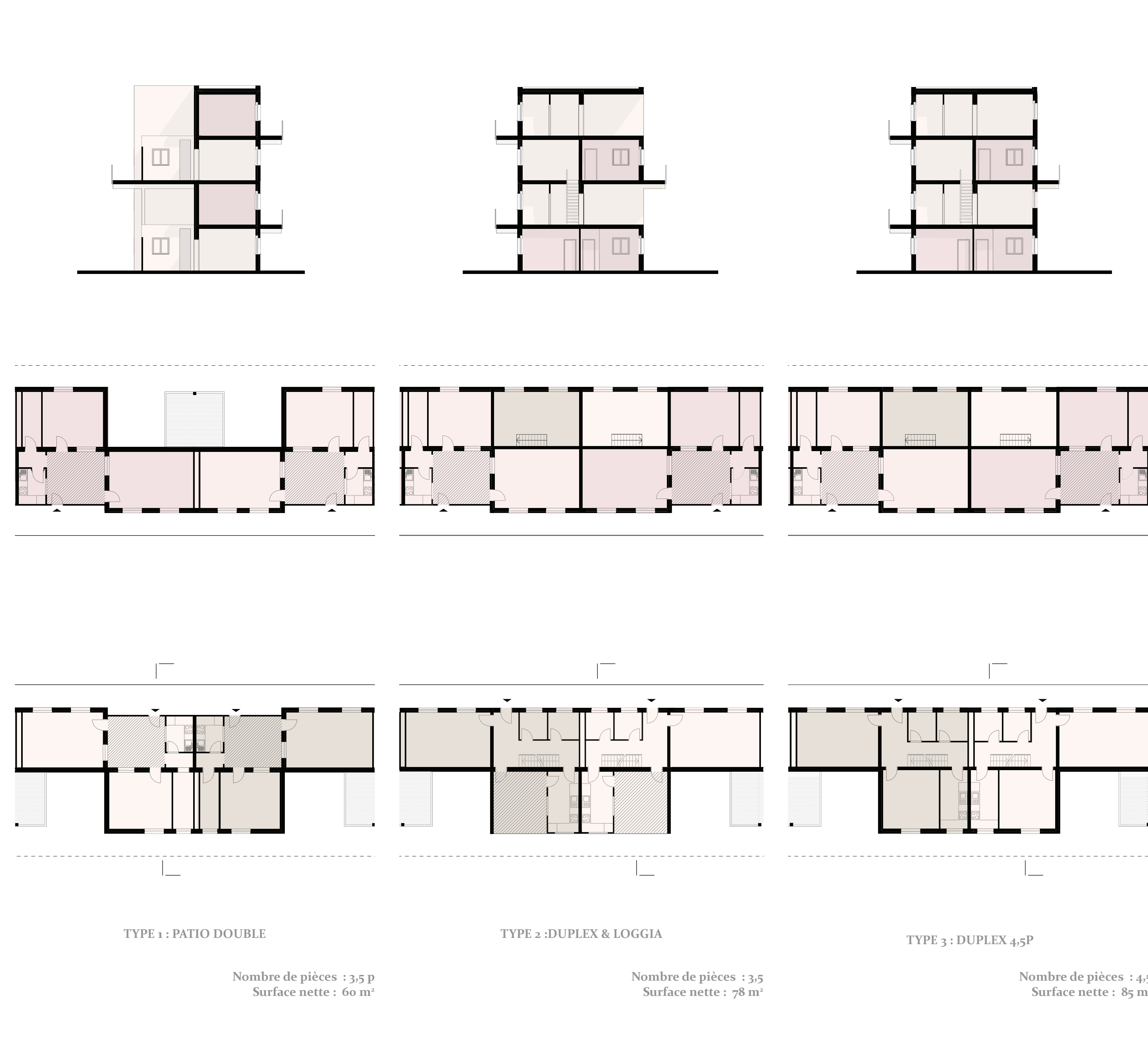
PLANS & COUPES TYPES 1:2000
