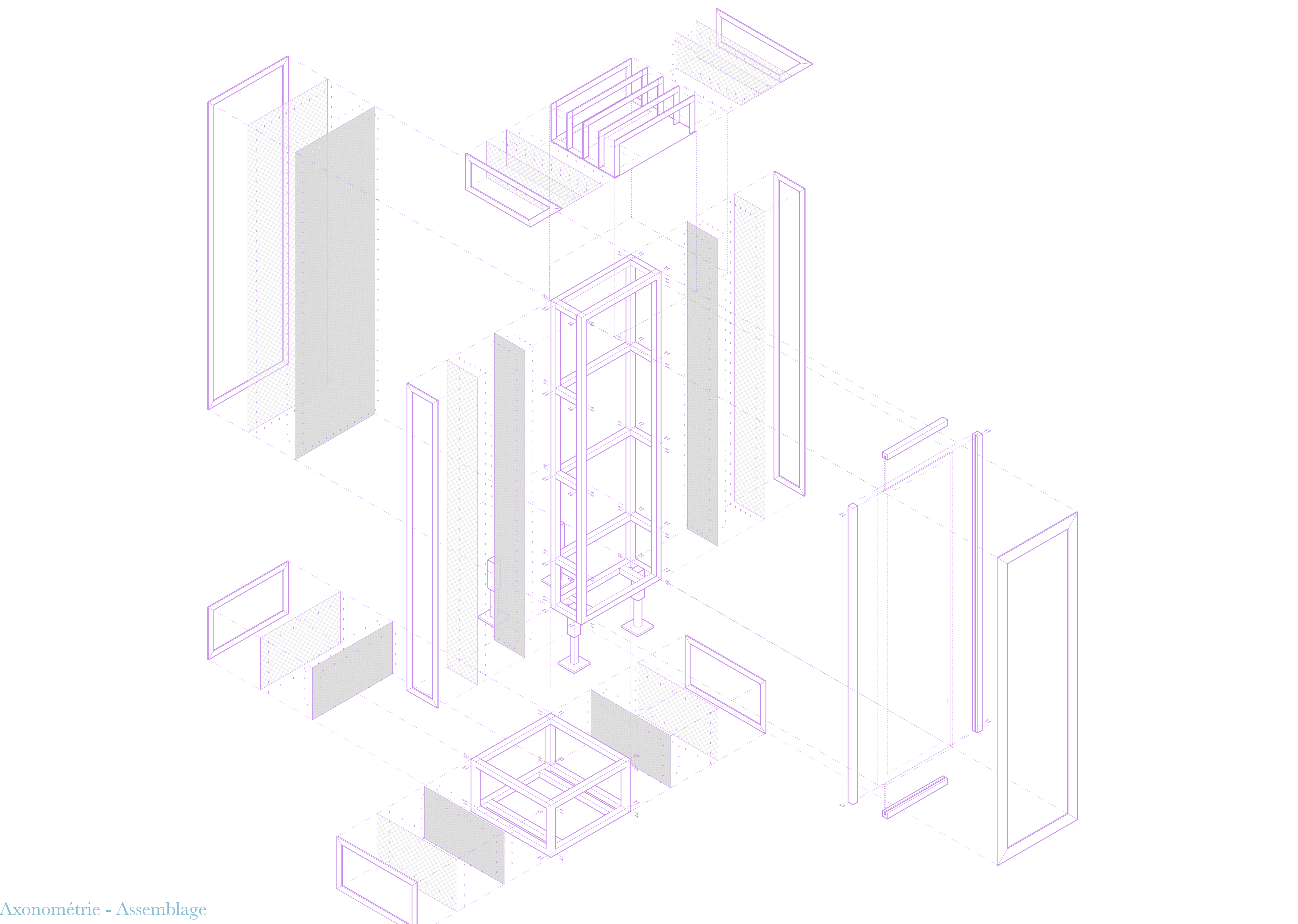
Axonométrie - Assemblage
