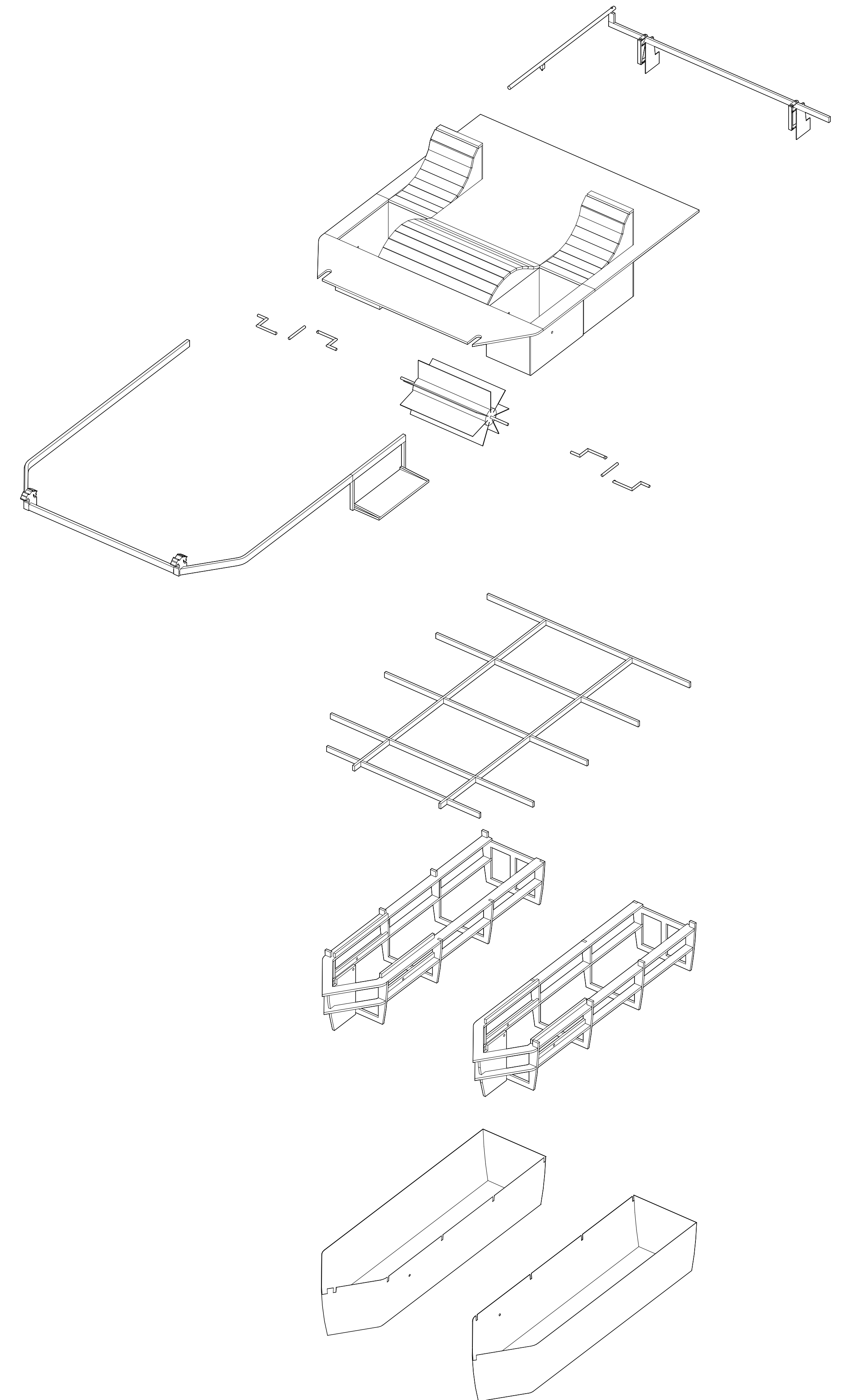
AXONOMÉTRIE ÉCLATÉE D'UN PÉDALO
