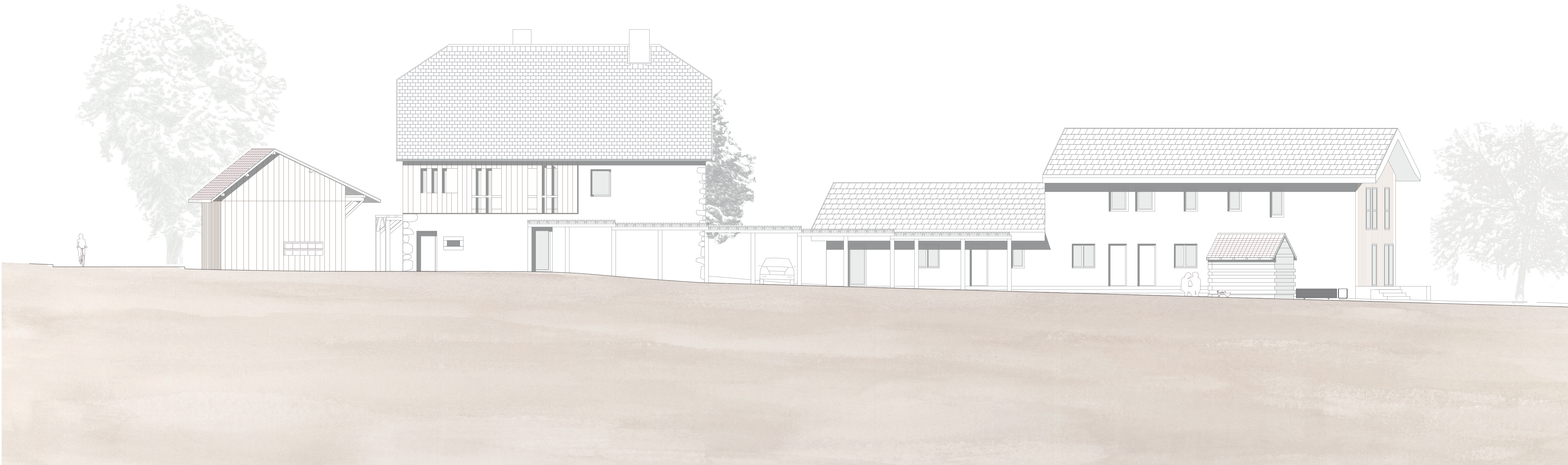
Section ee' 1:100
