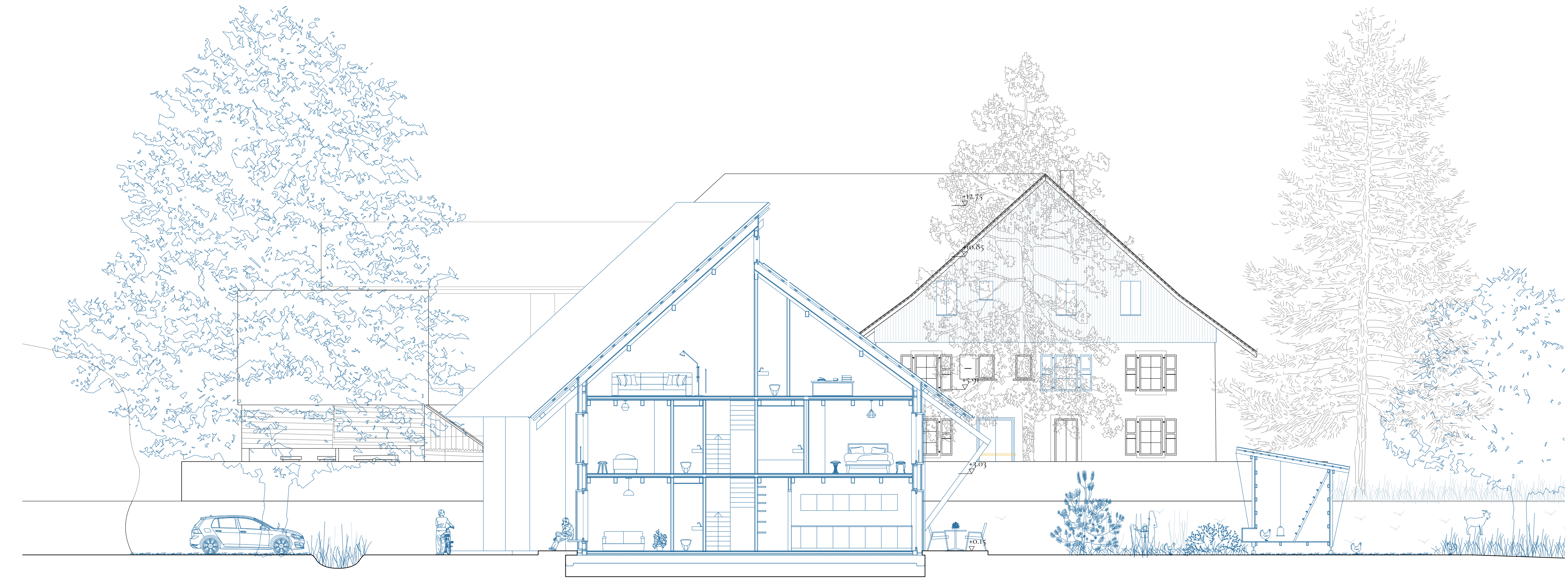
Coupe transversale | 1:100
