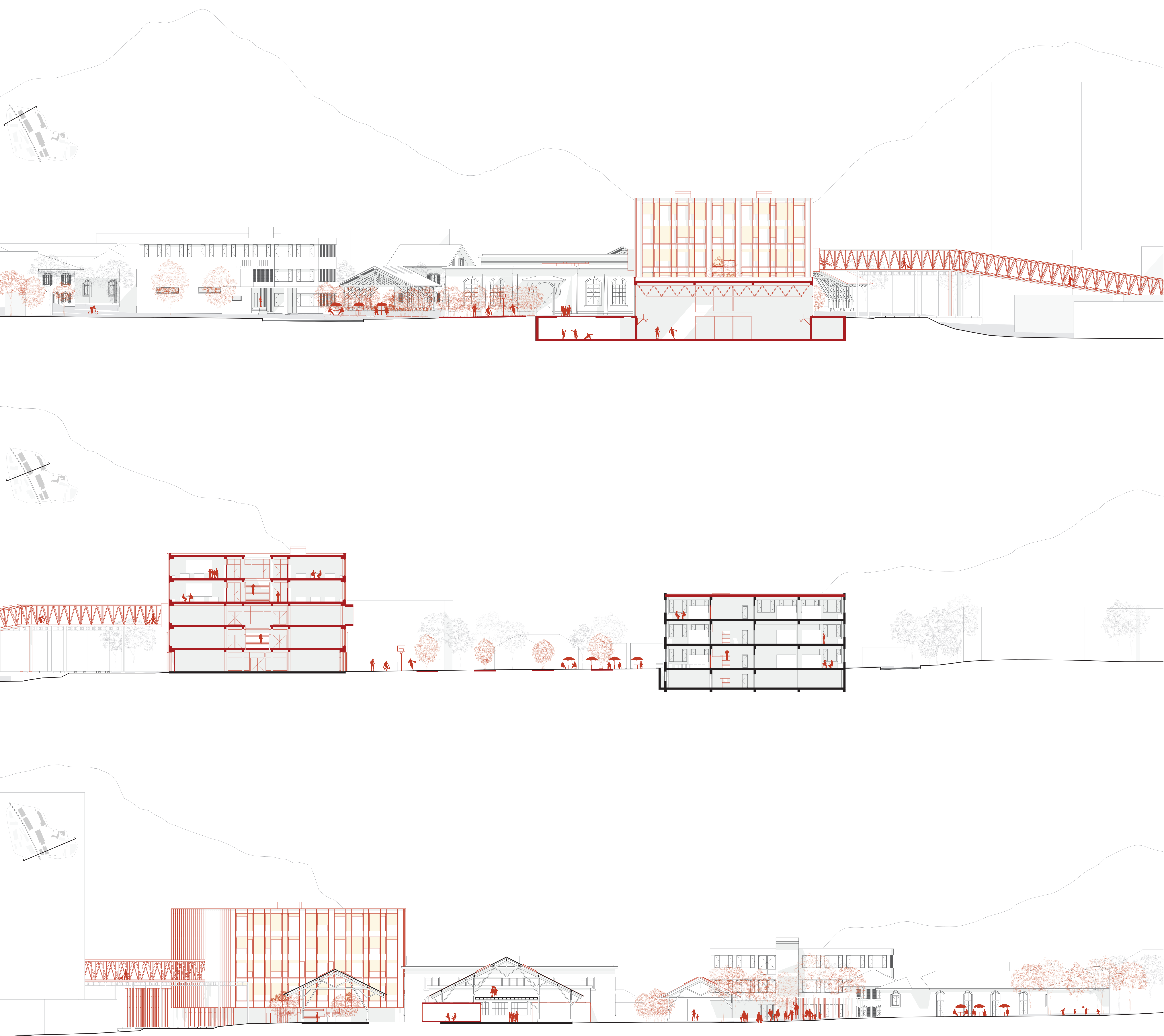
COUPES TRANSVERSALES 1:200
