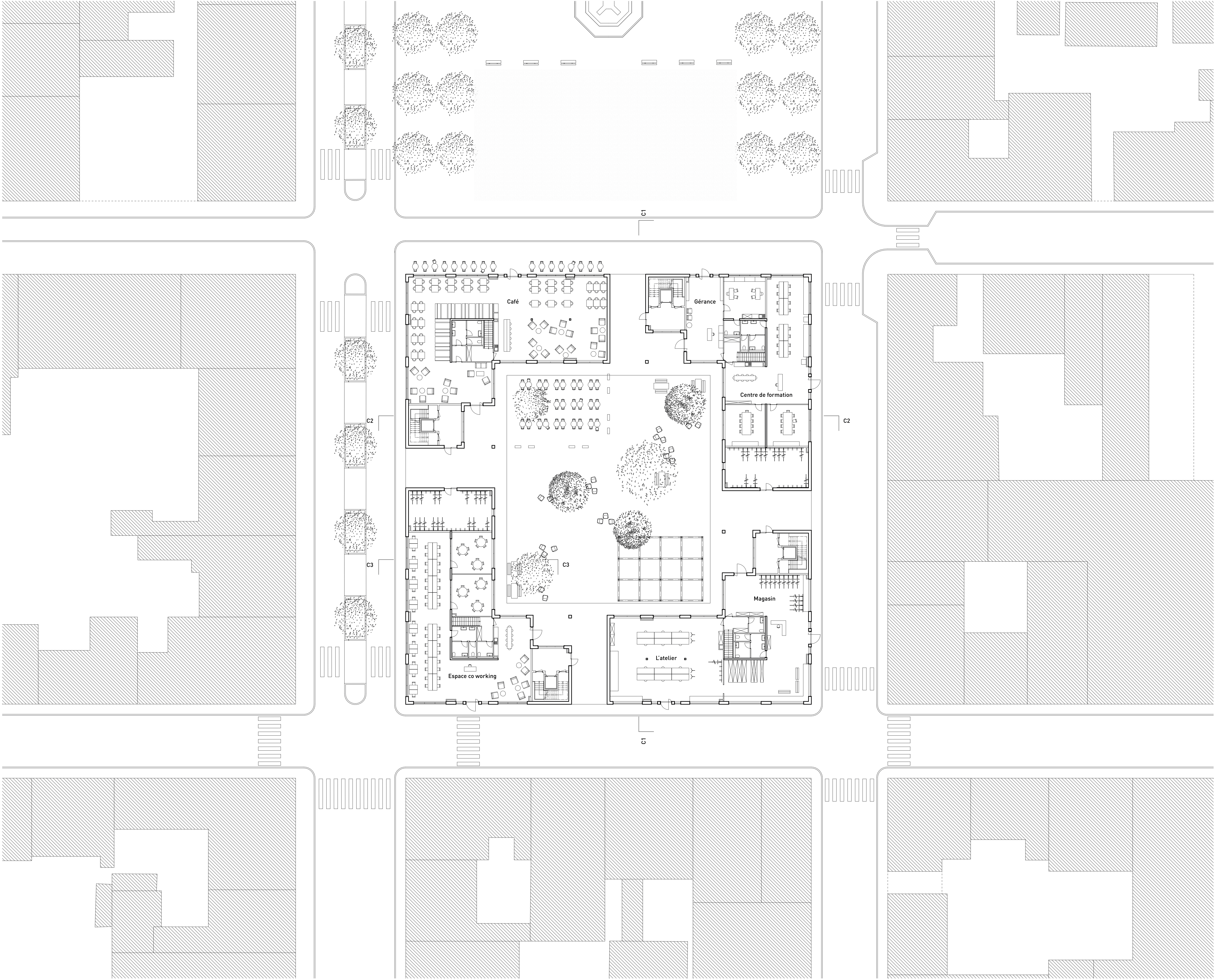
PLAN REZ-DE-CHAUSSEE E 1:200
