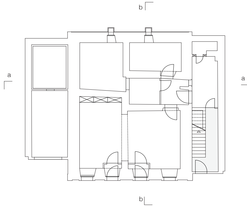
plan du rez-de-chaussée (2017)
