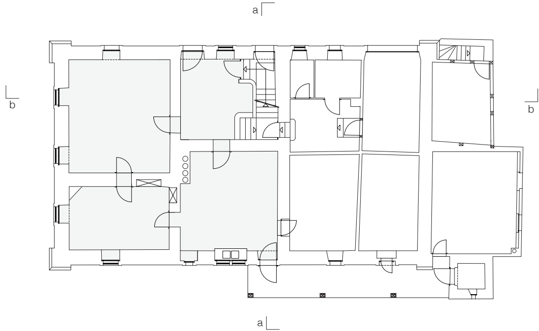
plan du rez-de-chaussée (2017)
