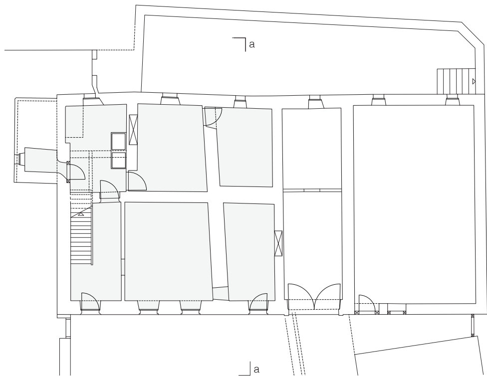
plan du rez-de-chaussée (1939)
