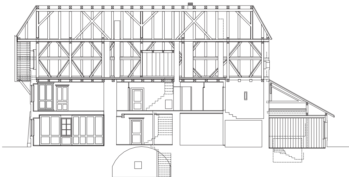
coupe b-b
