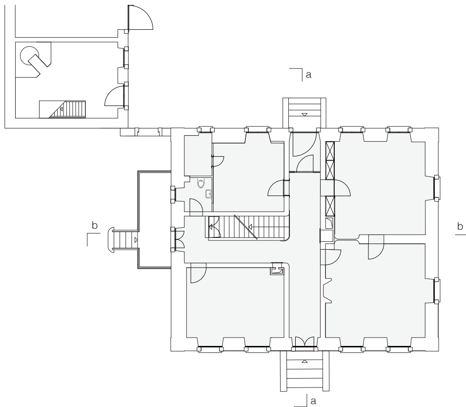
plan du rez-de-chaussée (2017)
