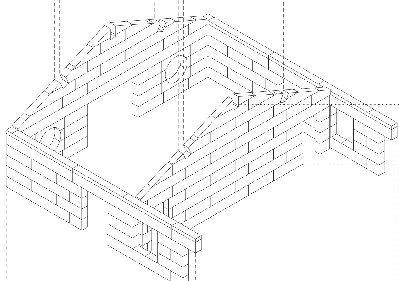
Appareillage en pierre massive locale : 150 cm x 35 cm x 60 cm
