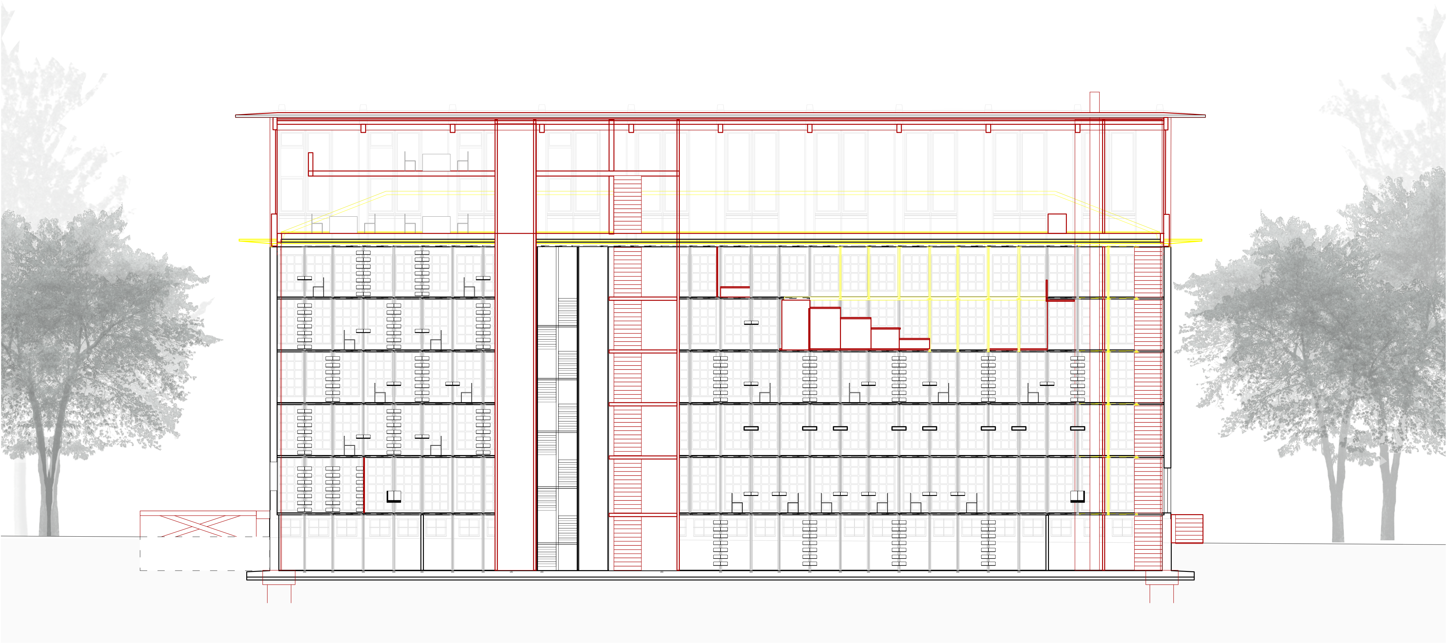
Coupe longitudinale 1:100
