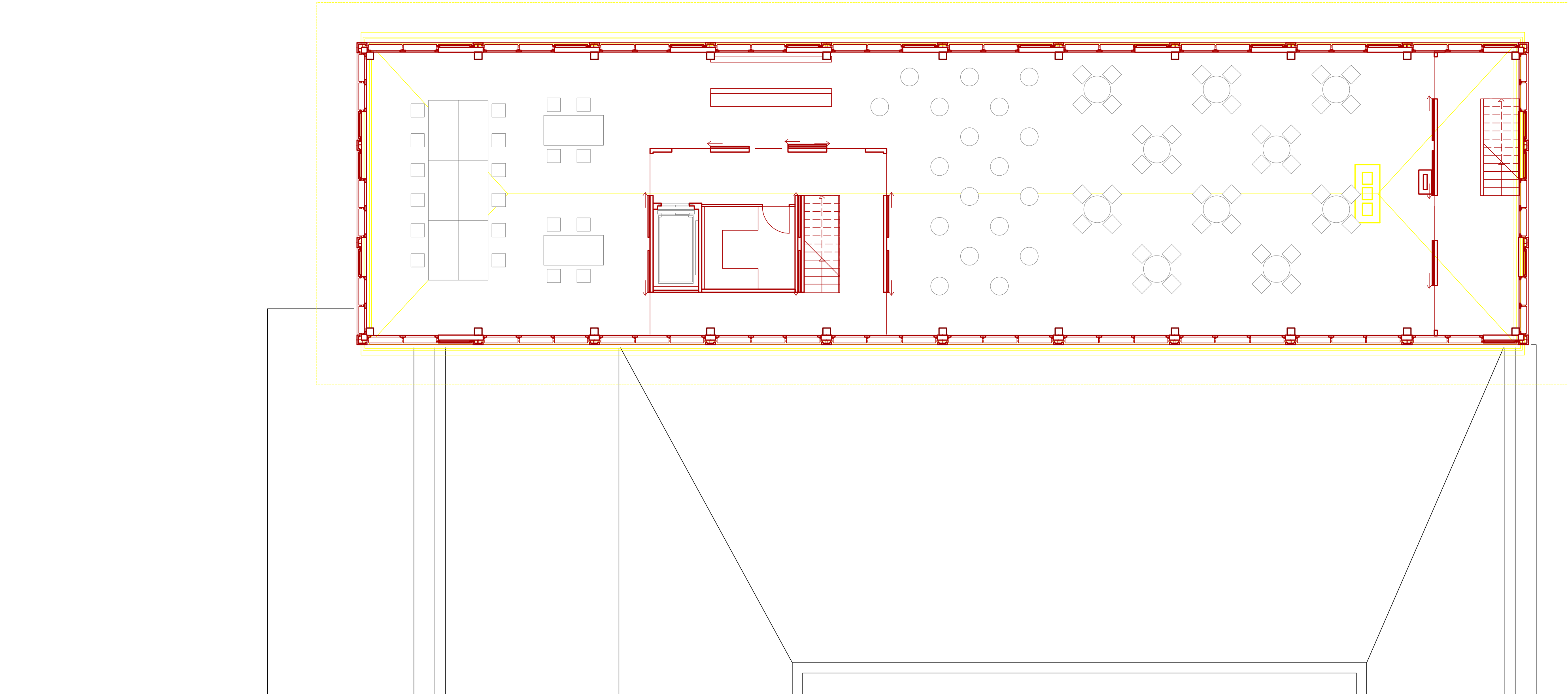
5. étage surélévation 1:100
