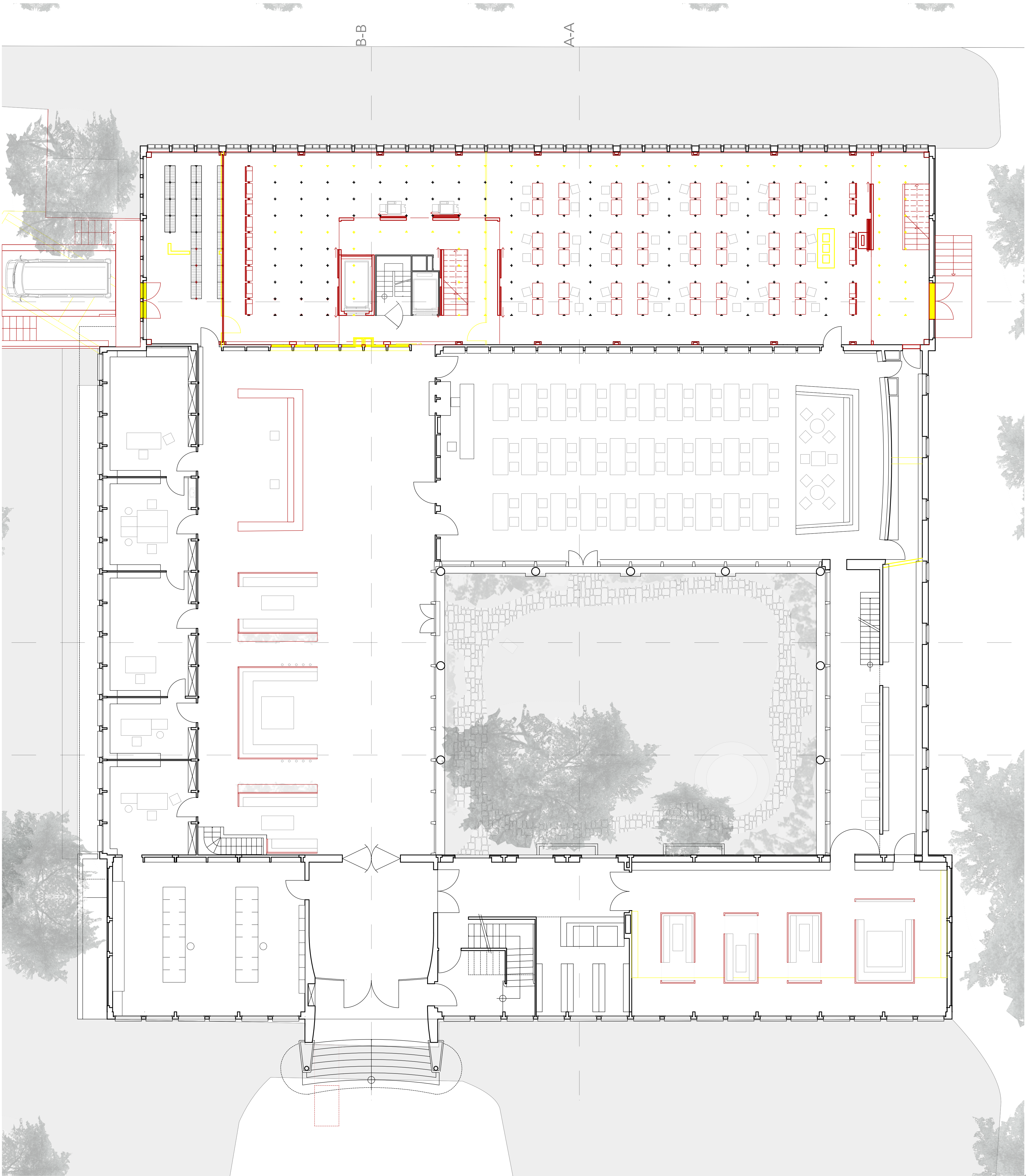
5. étage surélévation 1:100
