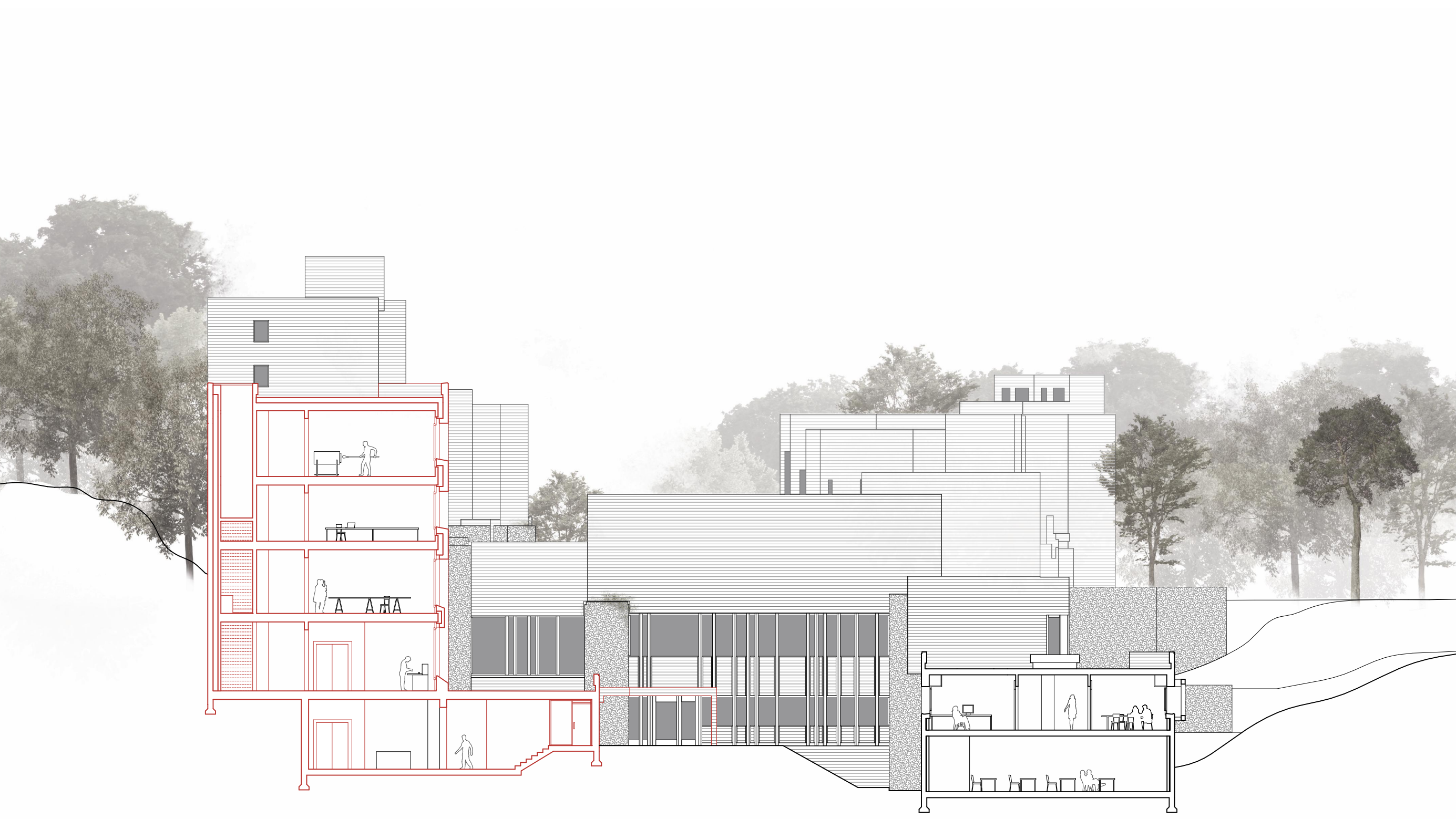
Coupe AA 1/200
