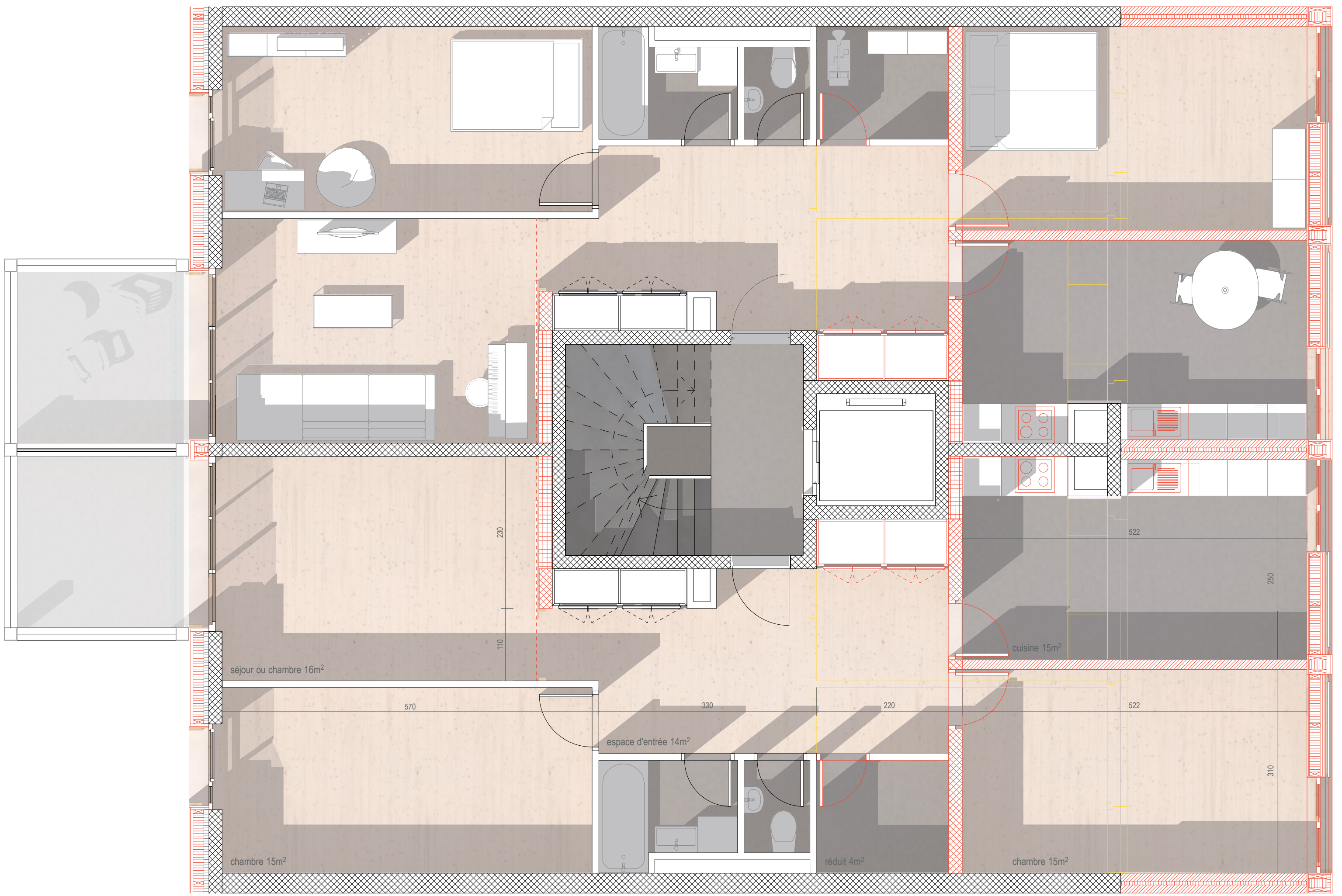
APPARTEMENT TYPE EXTENSION_1:50
