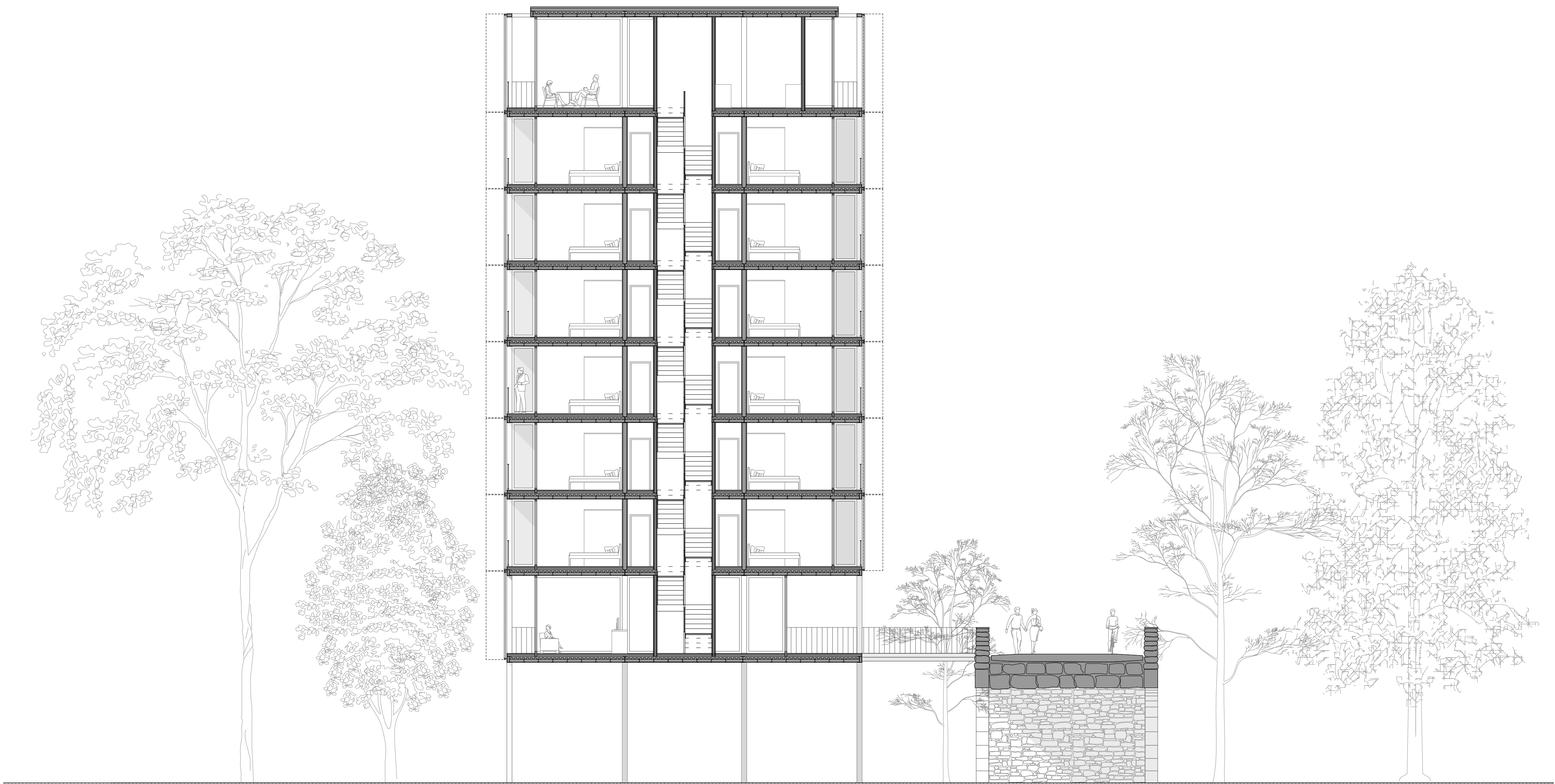
Coupe A-A 1:100
