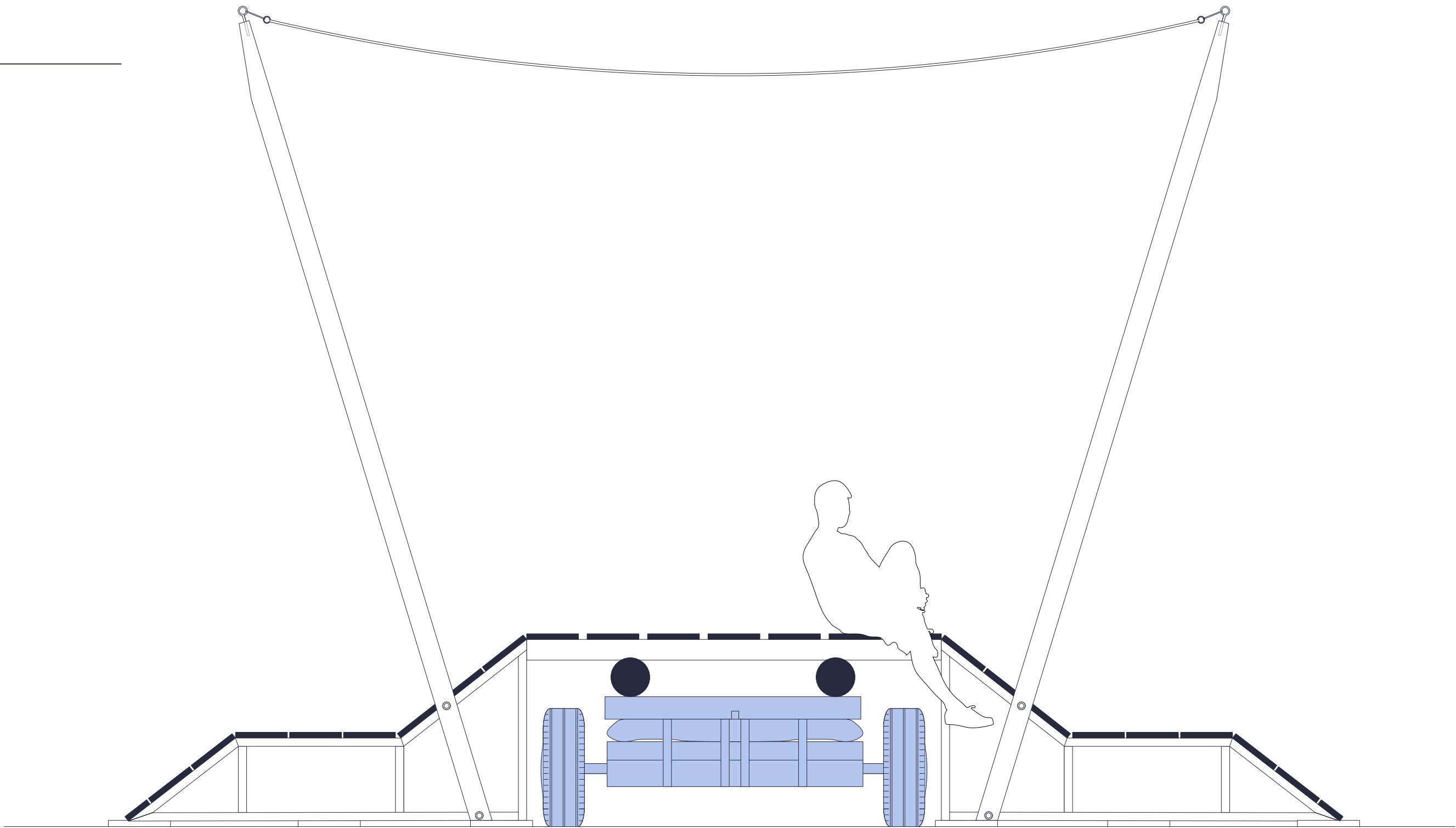
GRADINS COUPE 1:20
