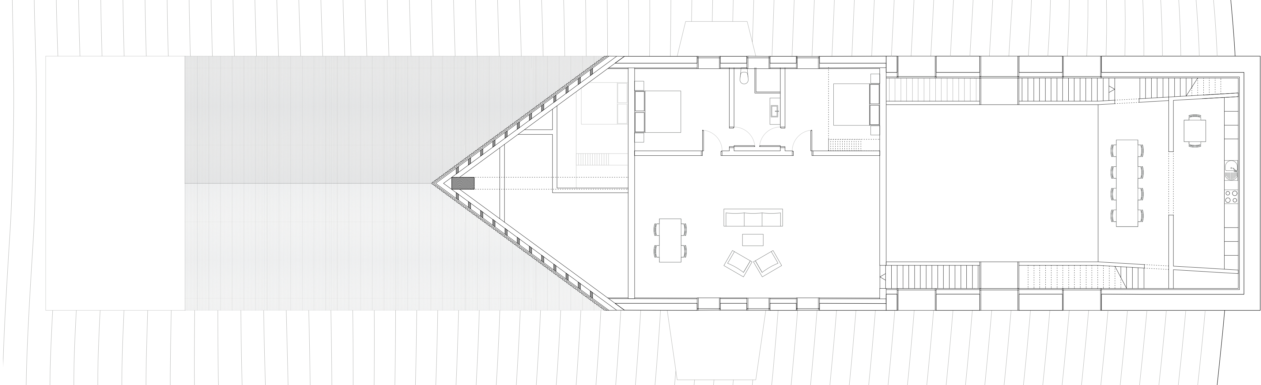
Plan appartement gardien / espace alpinistes 1:100
