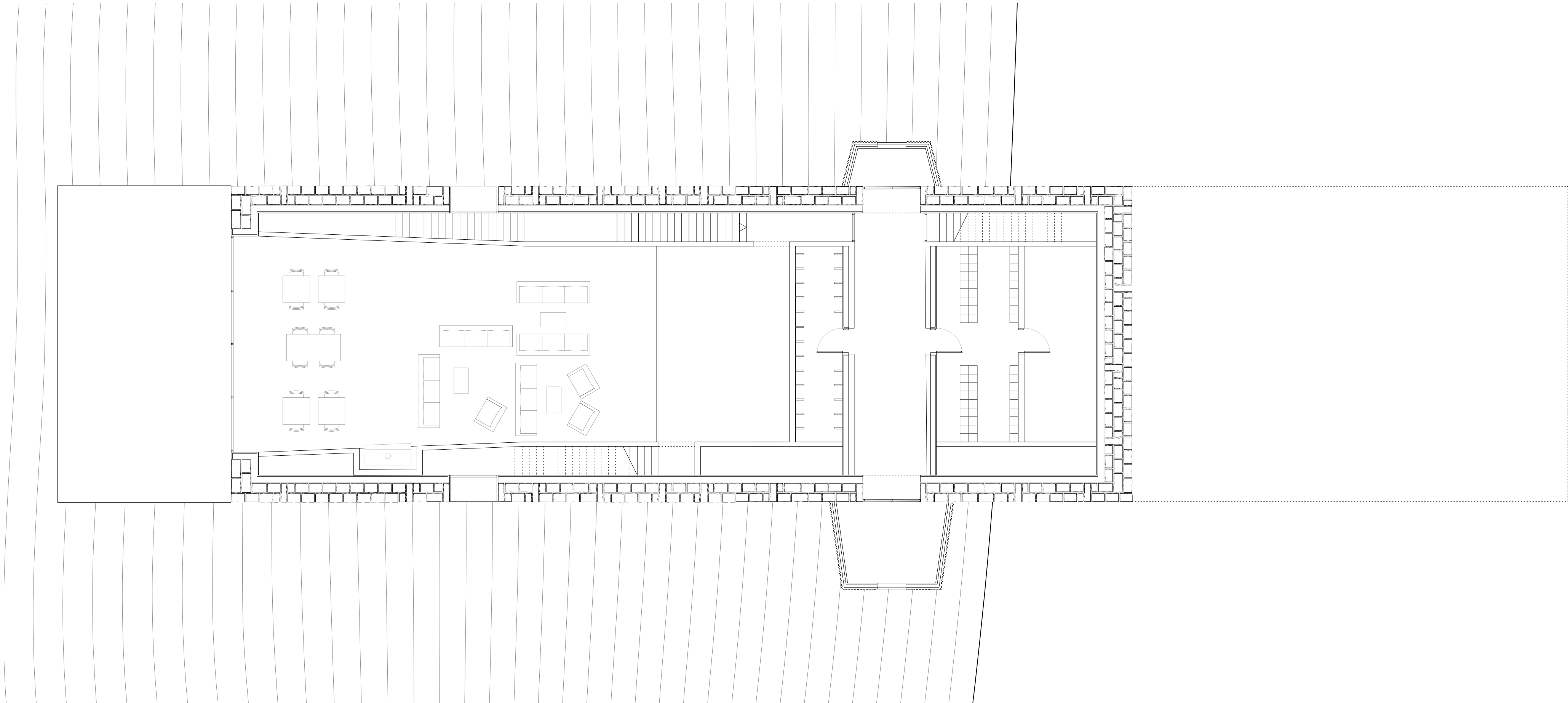
Plan entrée 1:100
