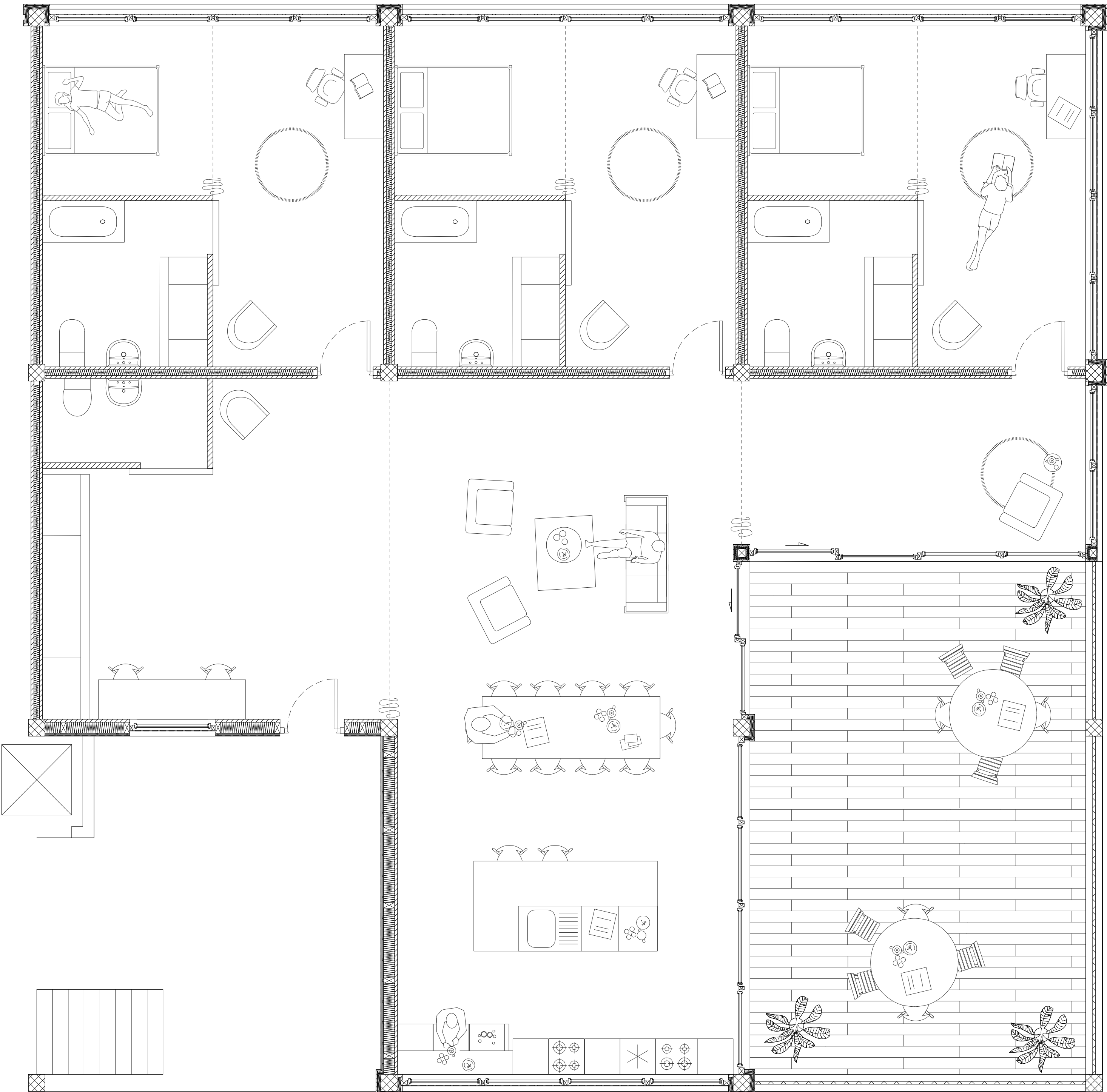
Plan d'étage type 1/200
