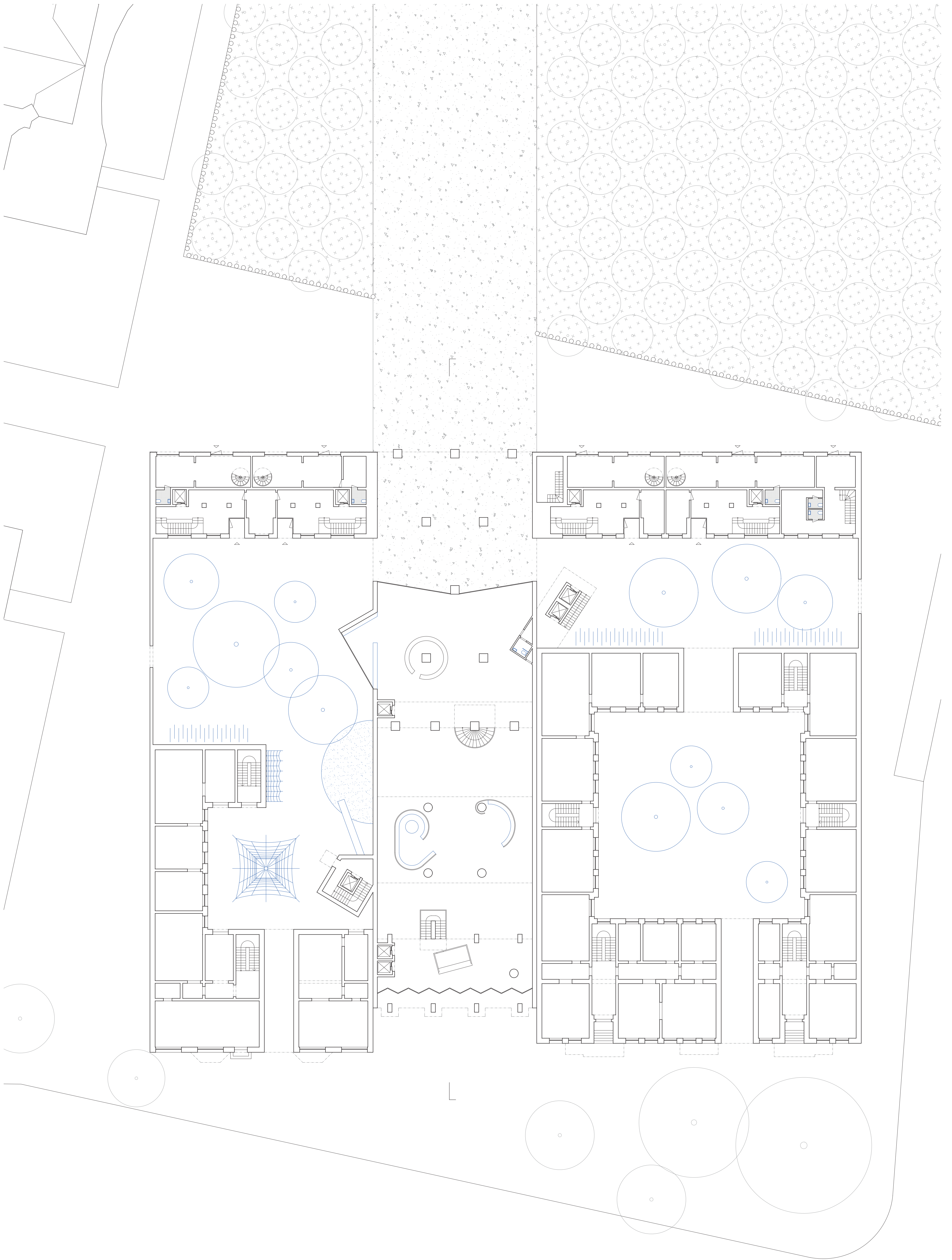
plan du rez-de-chaussée, 1:200
