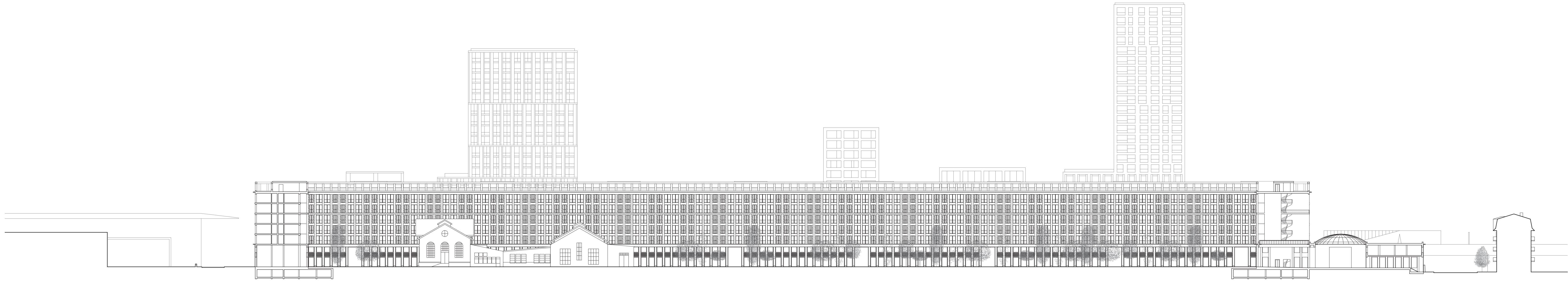
Coupe longitudinale AA' - 1:500
