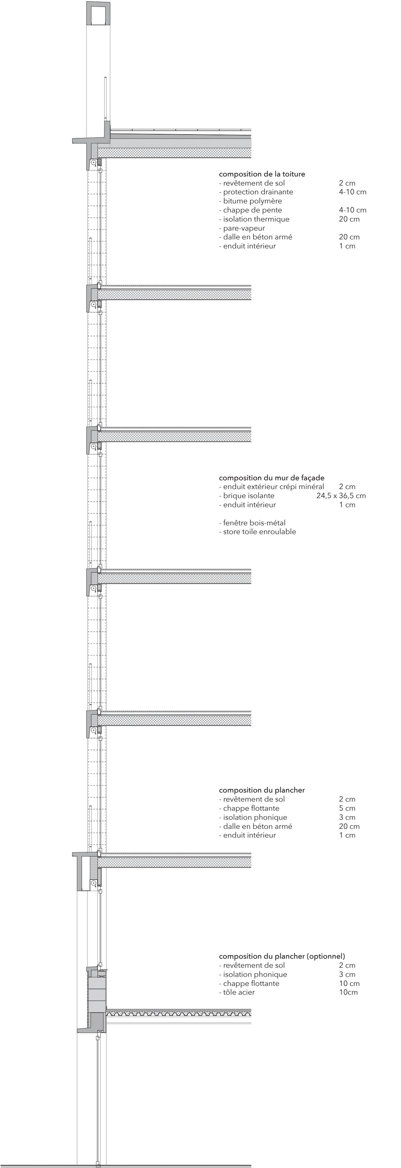
Coupe constructive - 1:50
