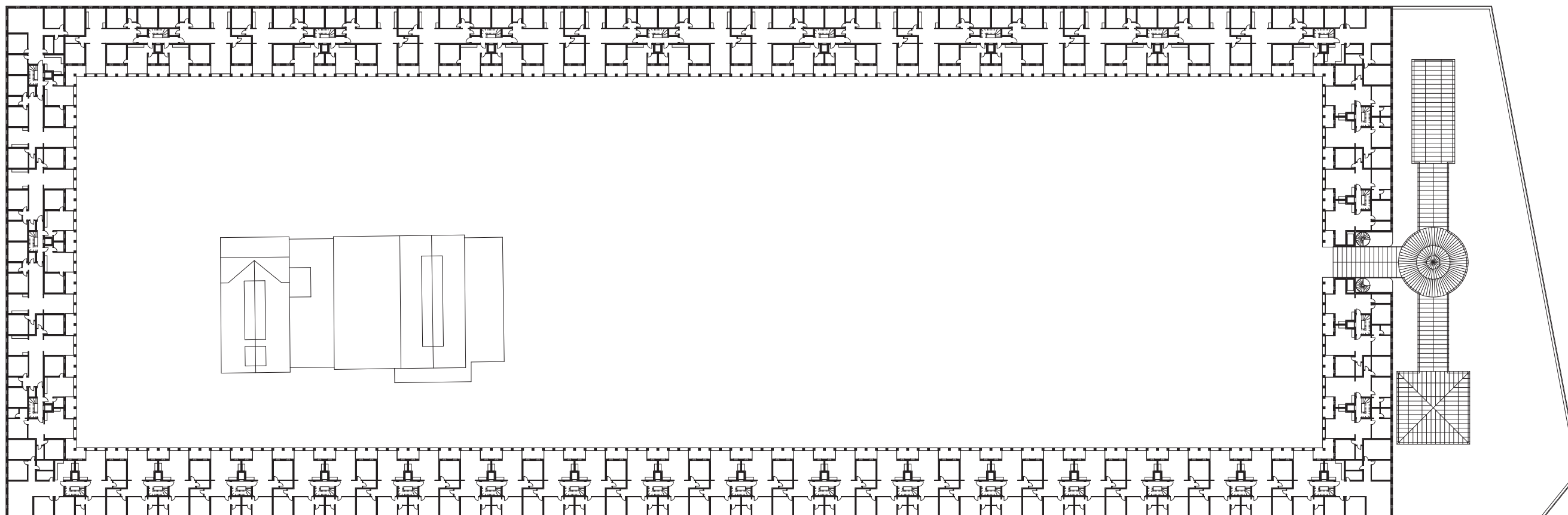
Plan étage type - 1:1'000
