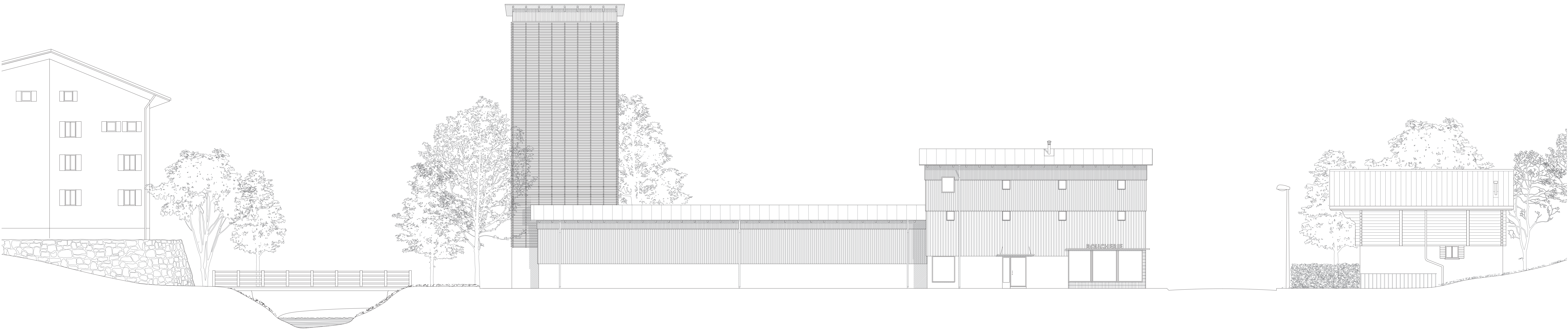
Elevation transversale B-B' -1/100 -
