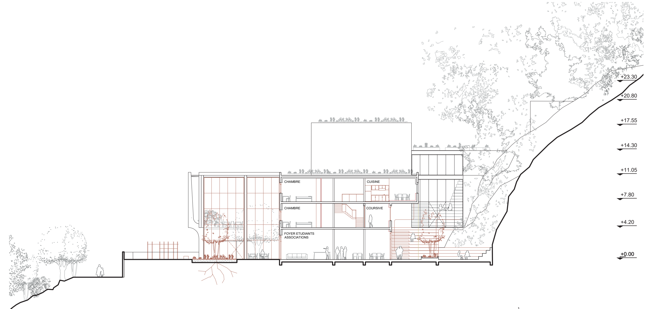
Coupe EE - Internat - Echelle 1:250
