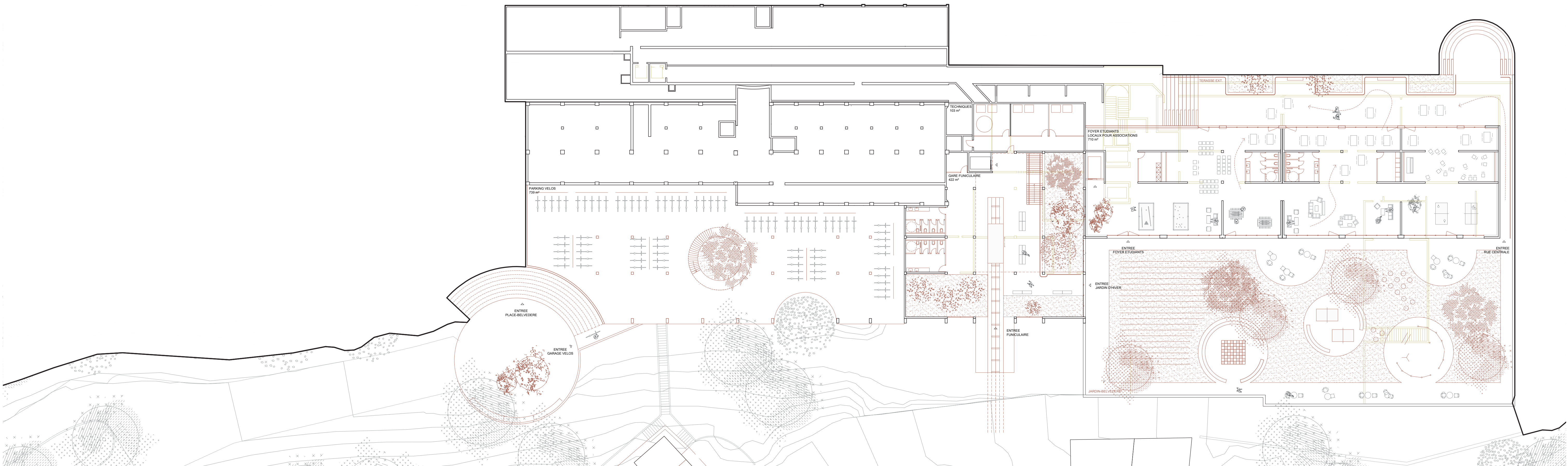
Niveau 0 - Echelle 1:250
