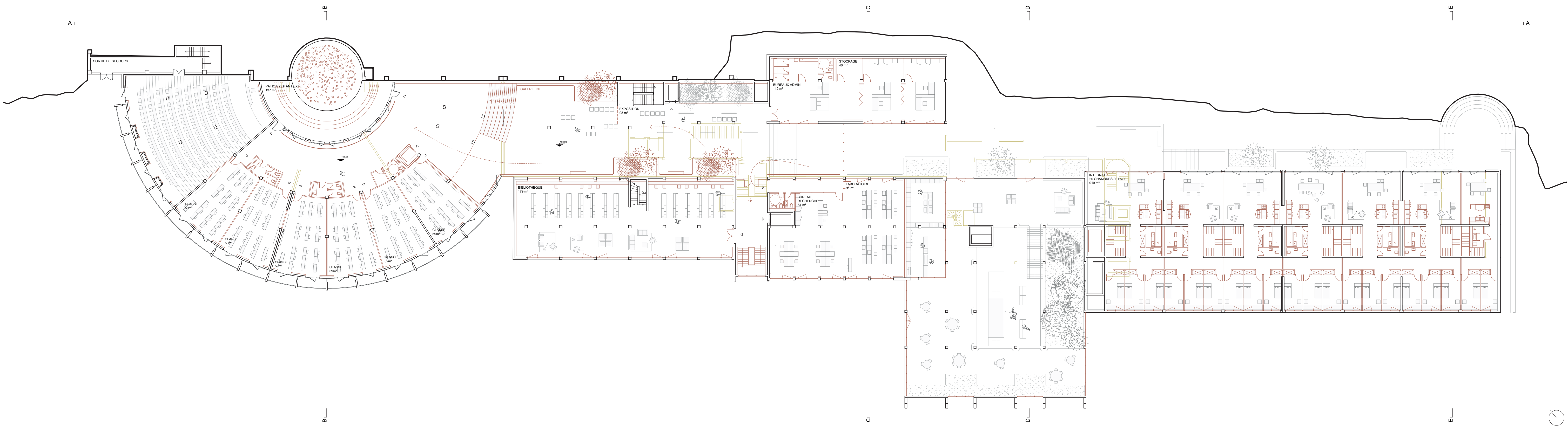
Niveau 2 - Echelle 1:250
