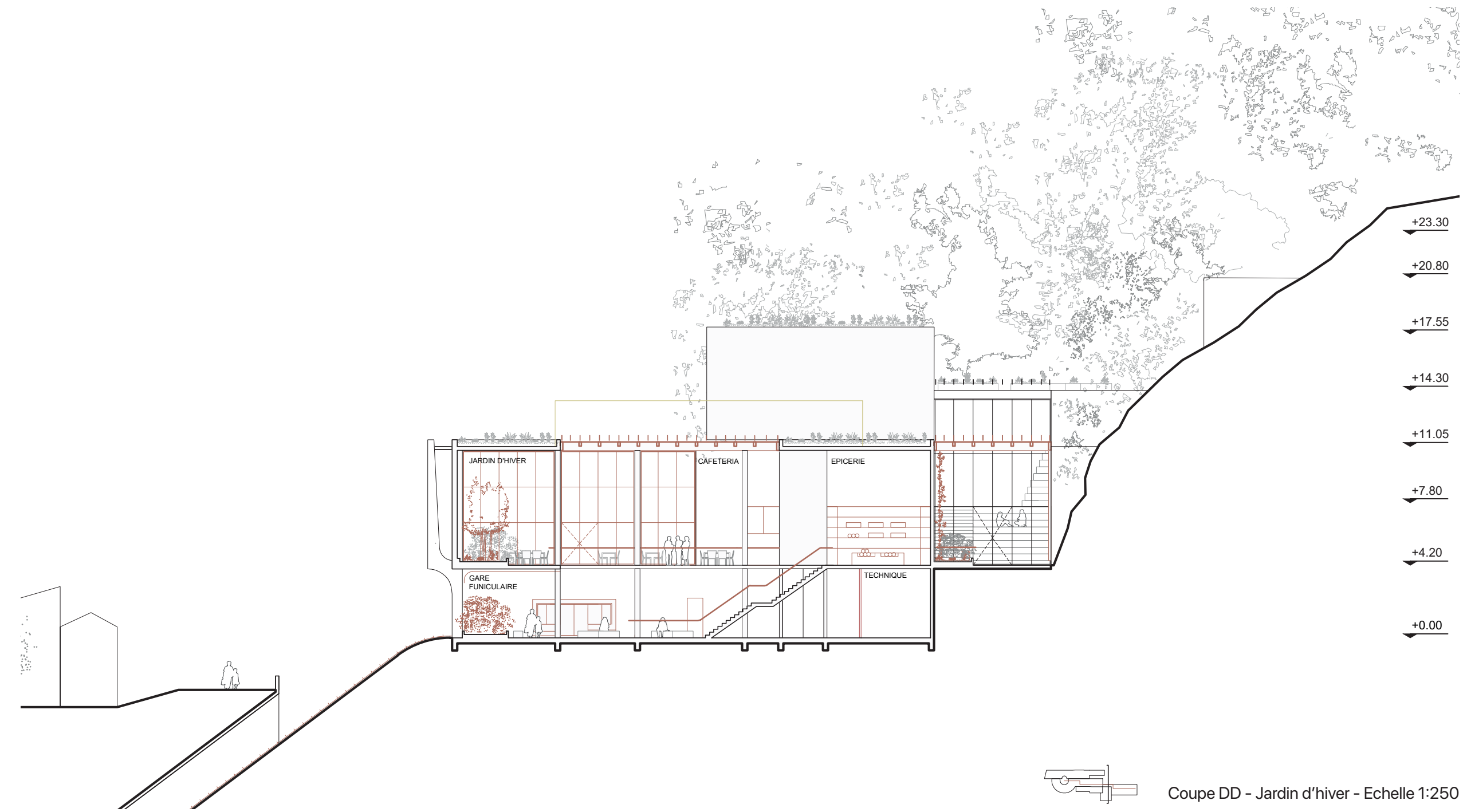
Coupe DD - Jardin d'hiver - Echelle 1:250
