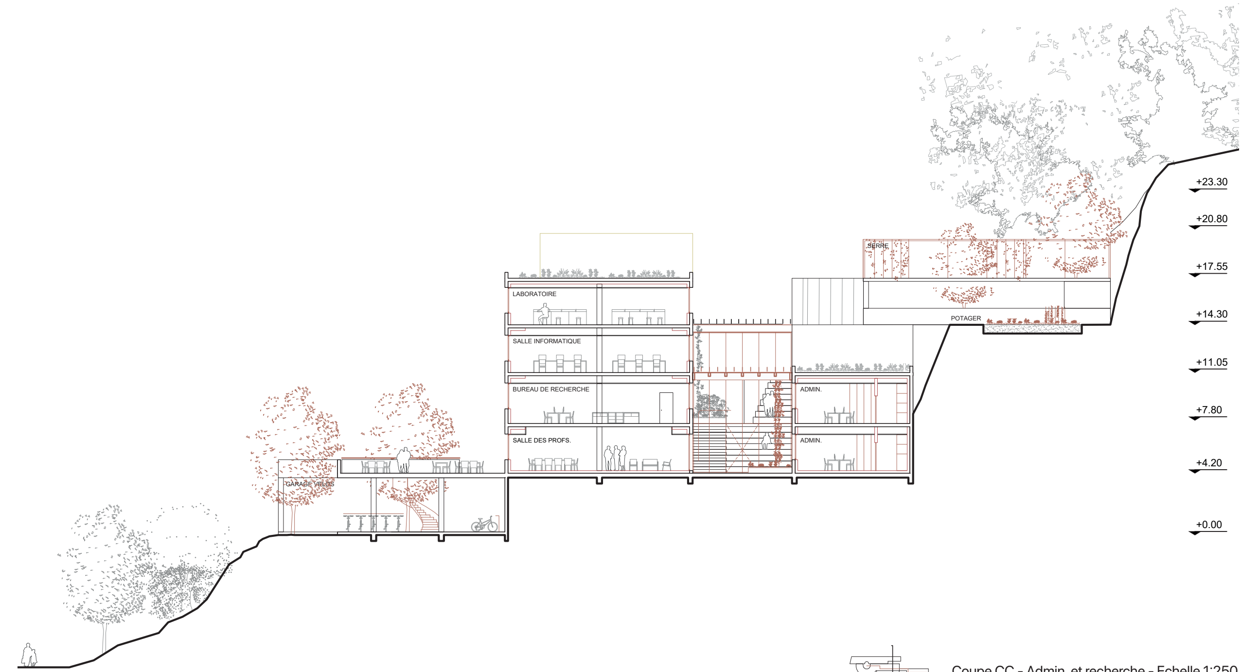
Coupe CC - Admin. et recherche - Echelle 1:250
