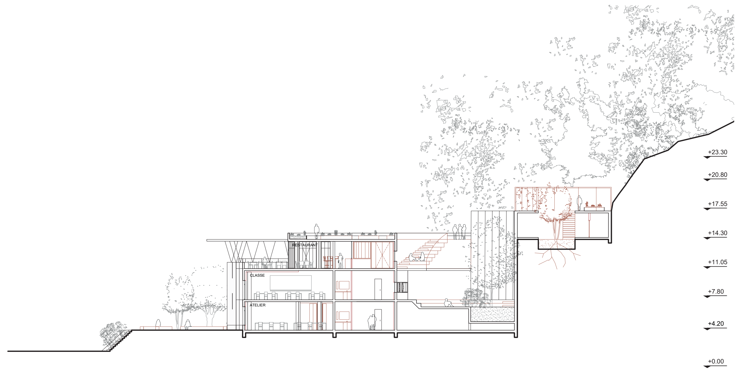
Coupe BB - Enseignement - Echelle 1:250
