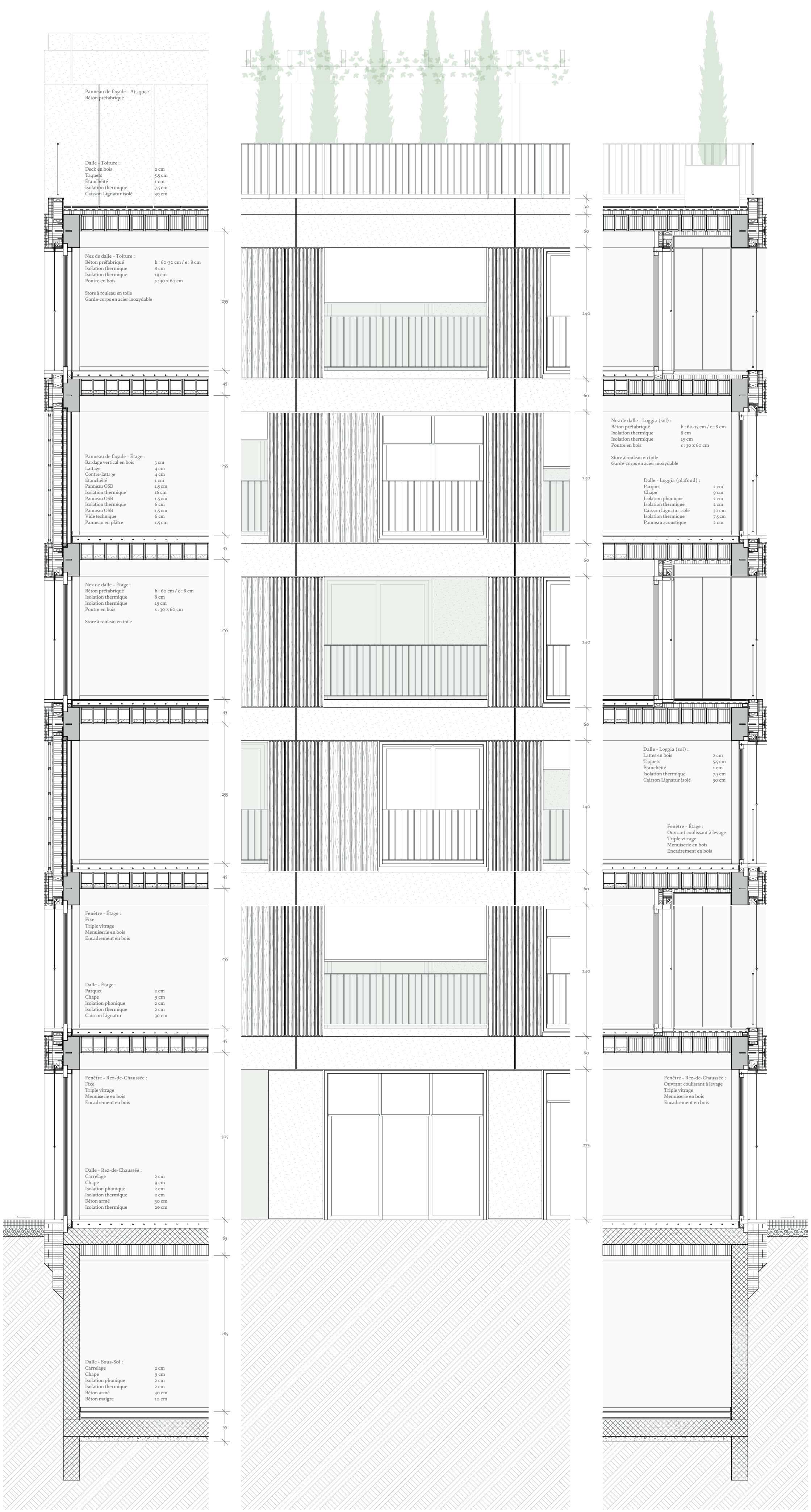
coupe constructive façade nord-est - 1:50
