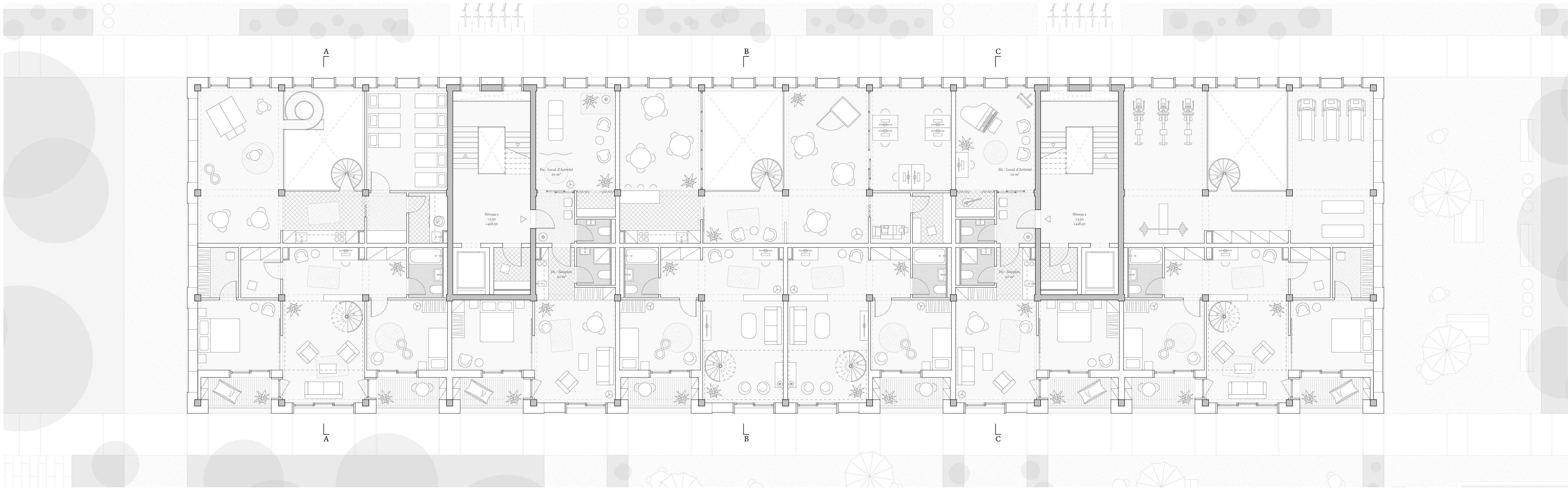
plan 1er étage - 1:100
