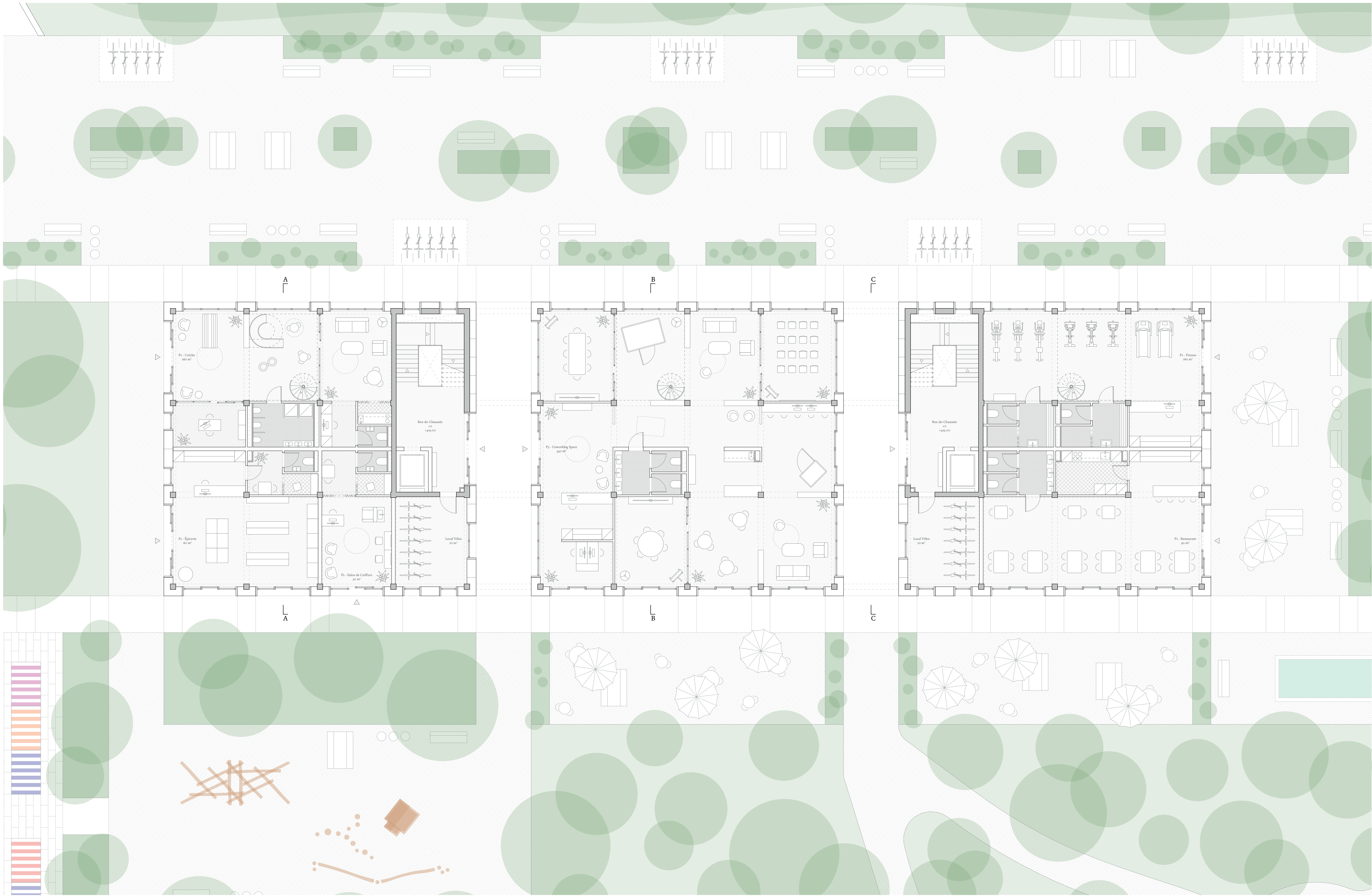
plan rez-de-chaussée - 1:100
