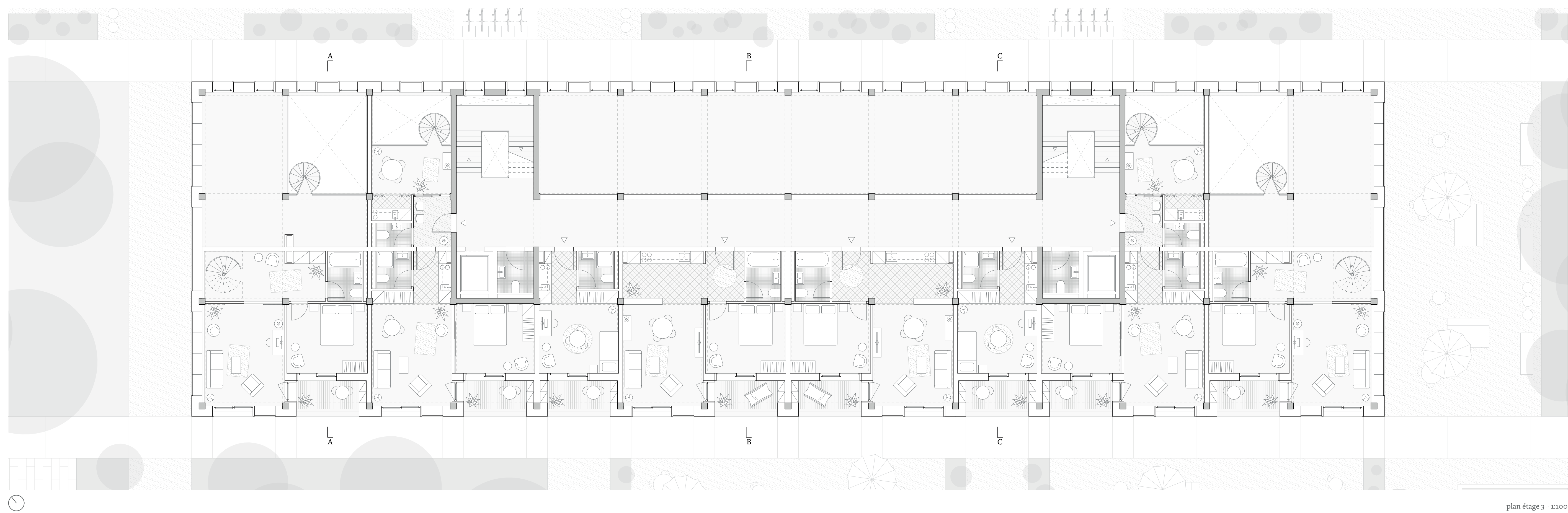
plan étage 3 - 1:100
