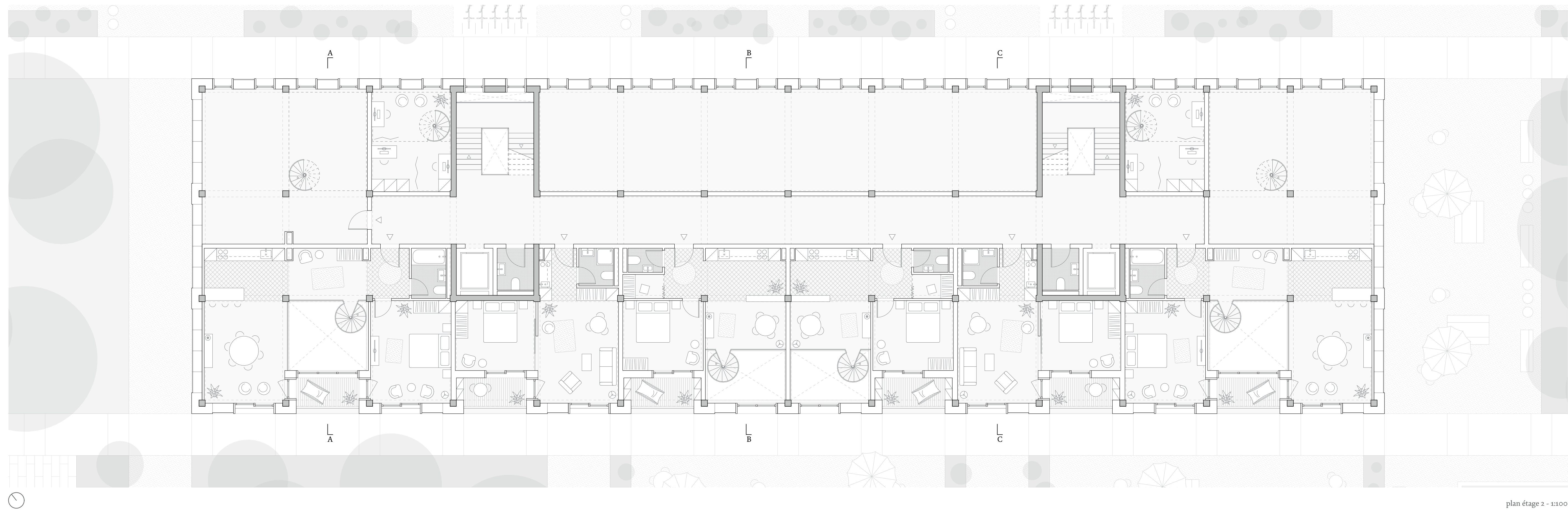
plan étage 2 - 1:100
