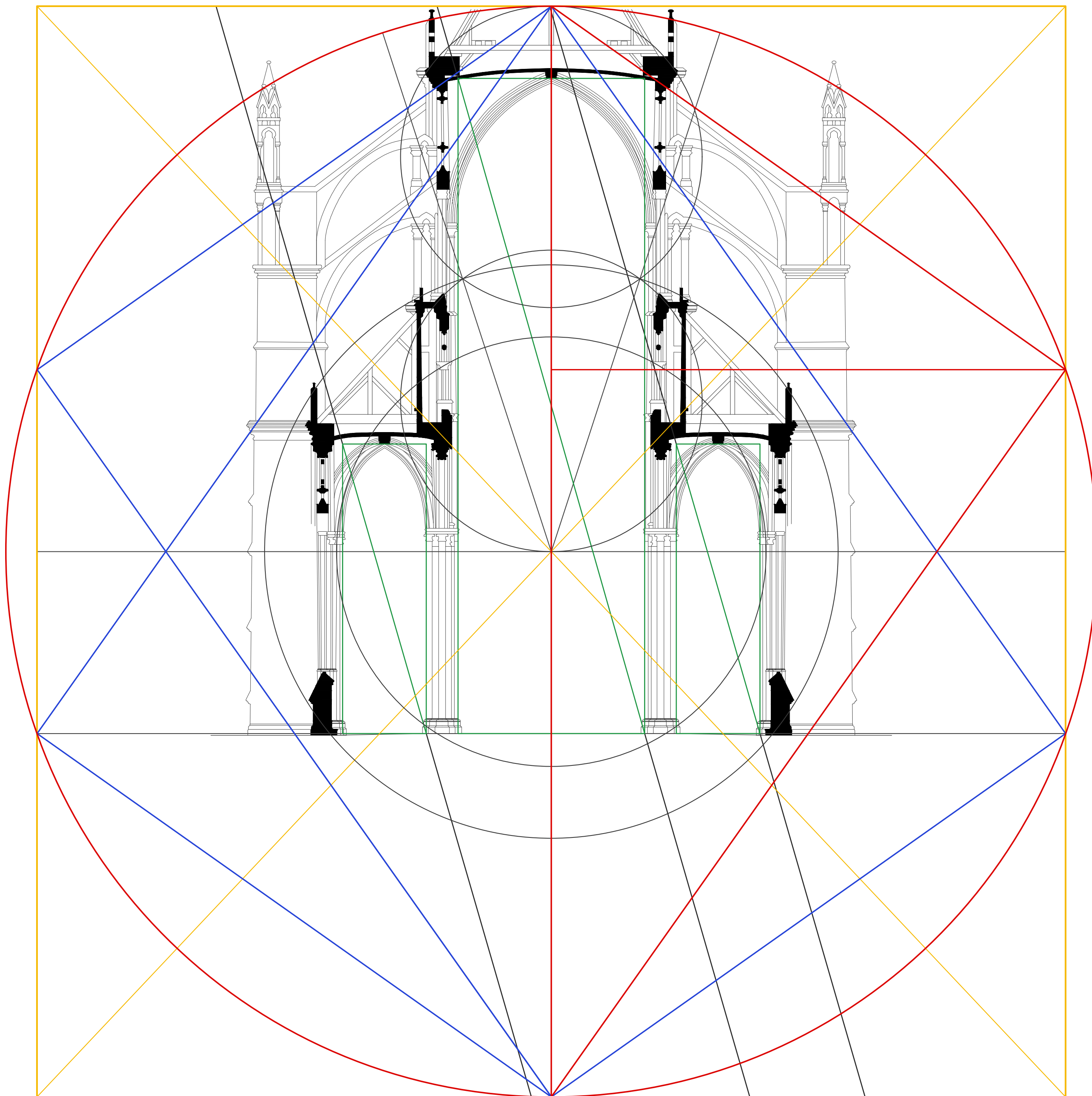
CATHEDRALE D'AMIENS Tracés proportionnels
