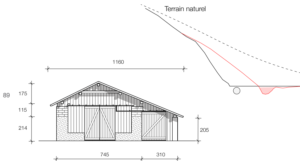
Façade Est; en rouge, le gabarit de la grange-écurie d'origine, une route en terre et un bisse. La route a été agrandie à l'arrivée de la voiture.
