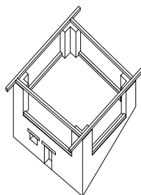
Entrails et sablières
