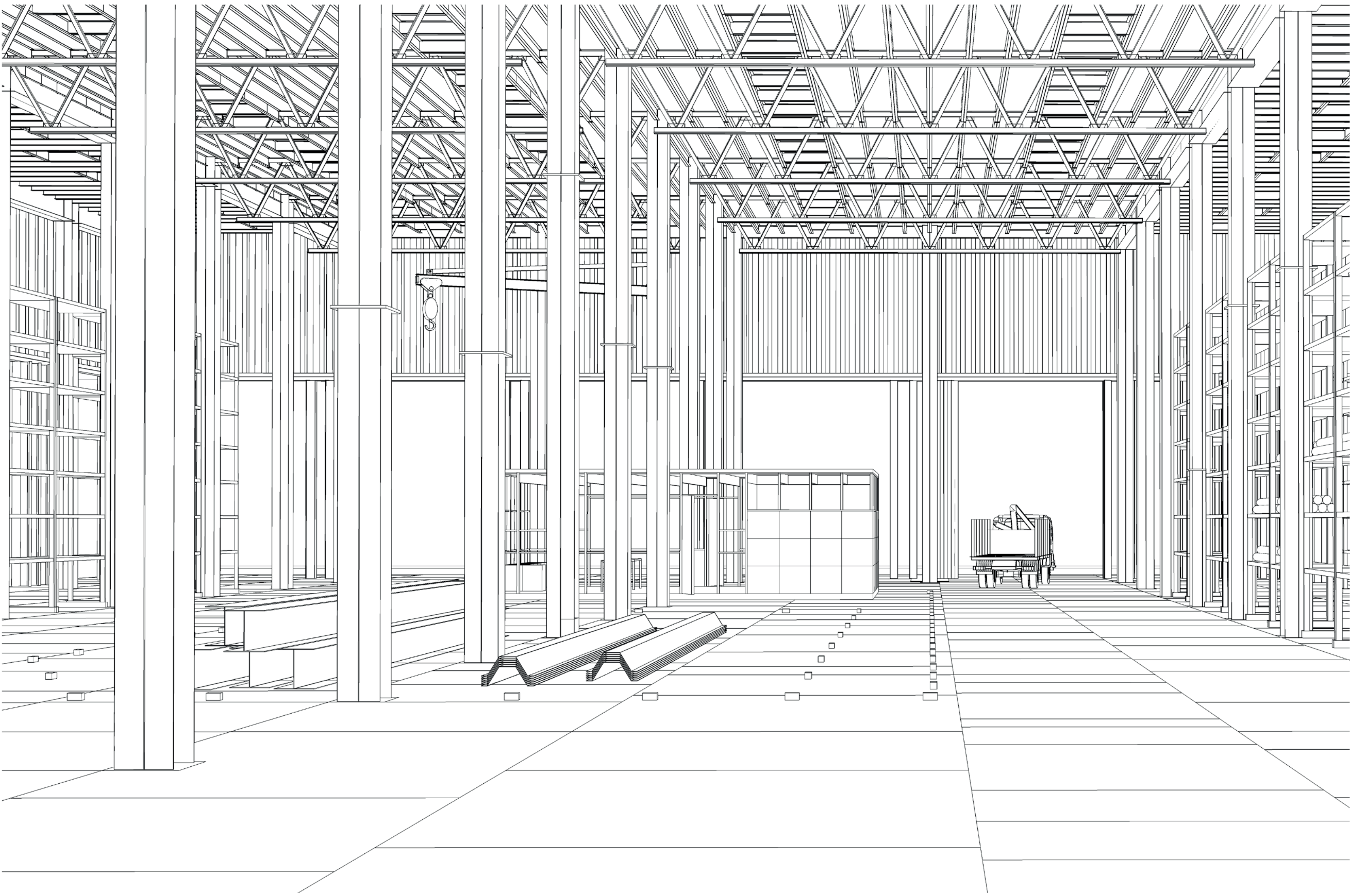
Perspective sur les espaces de travail pour éléments XL derrière la façade flexible
