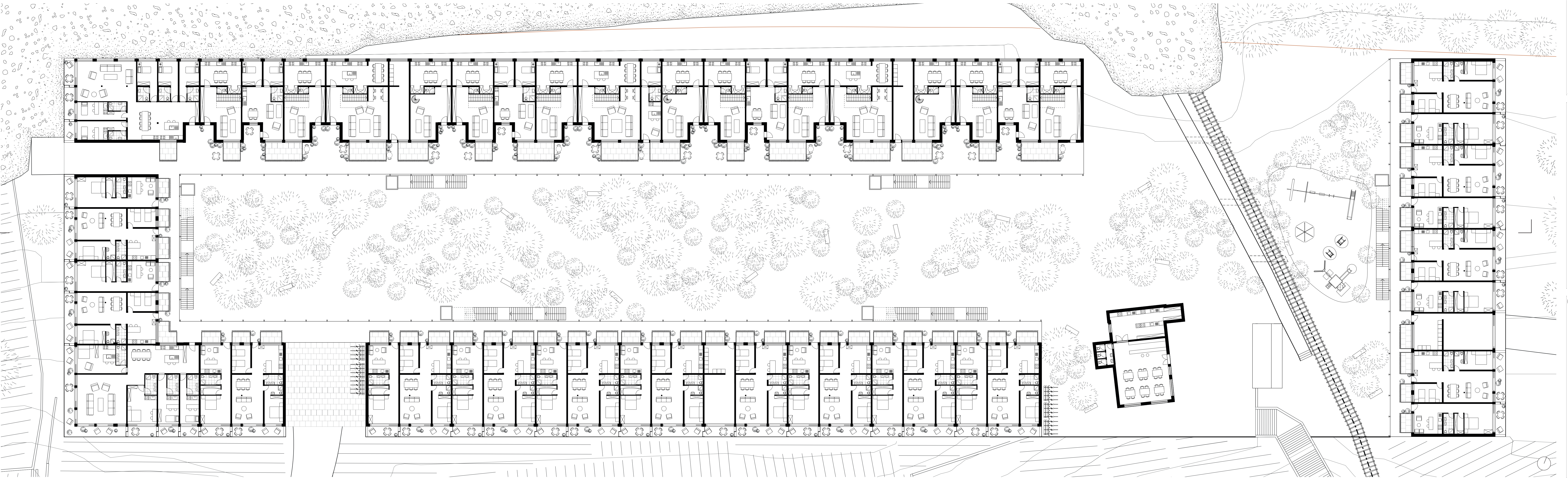
Plan de premier étage 1:200
