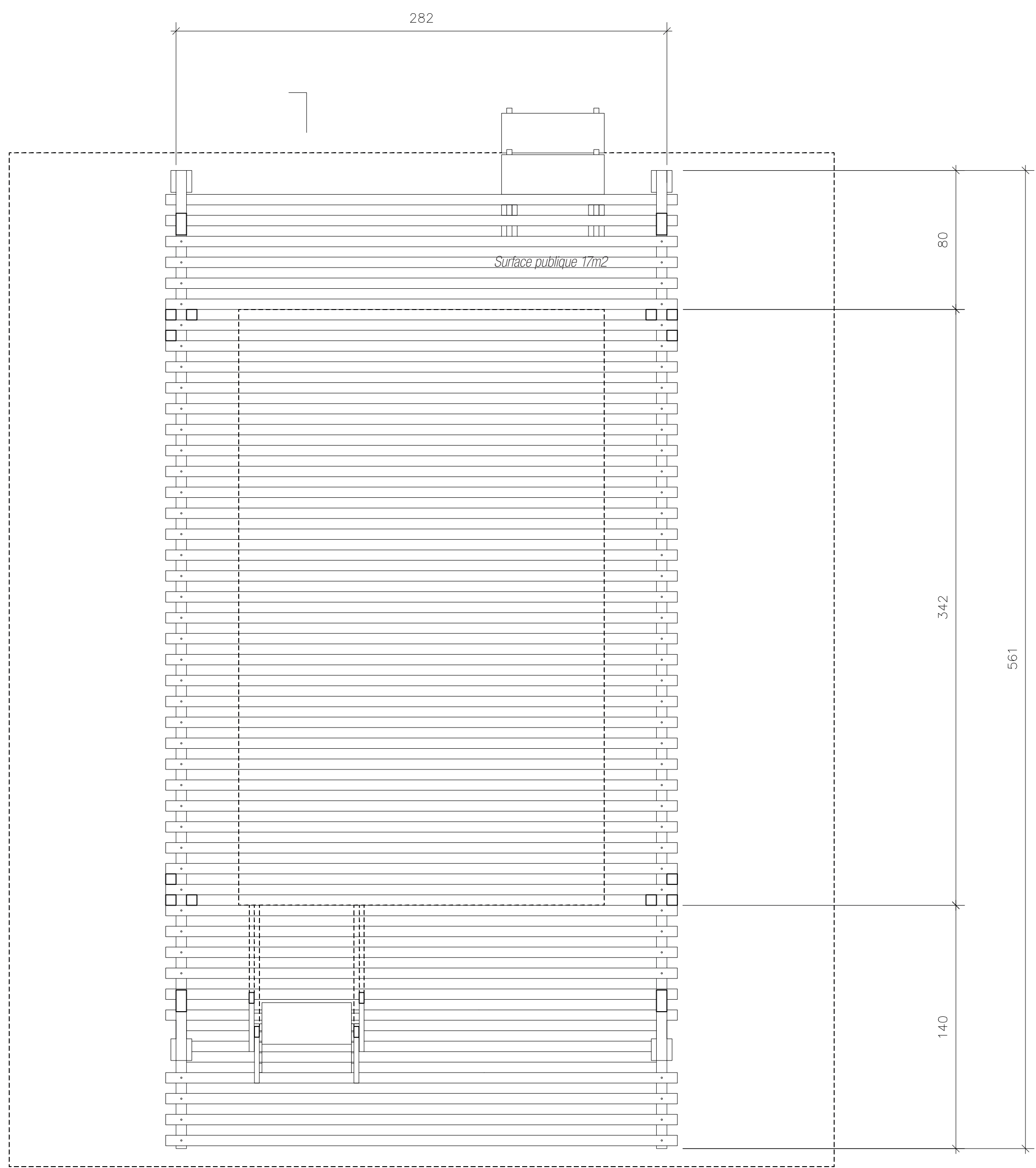
Plan niveau inférieur 1.20
