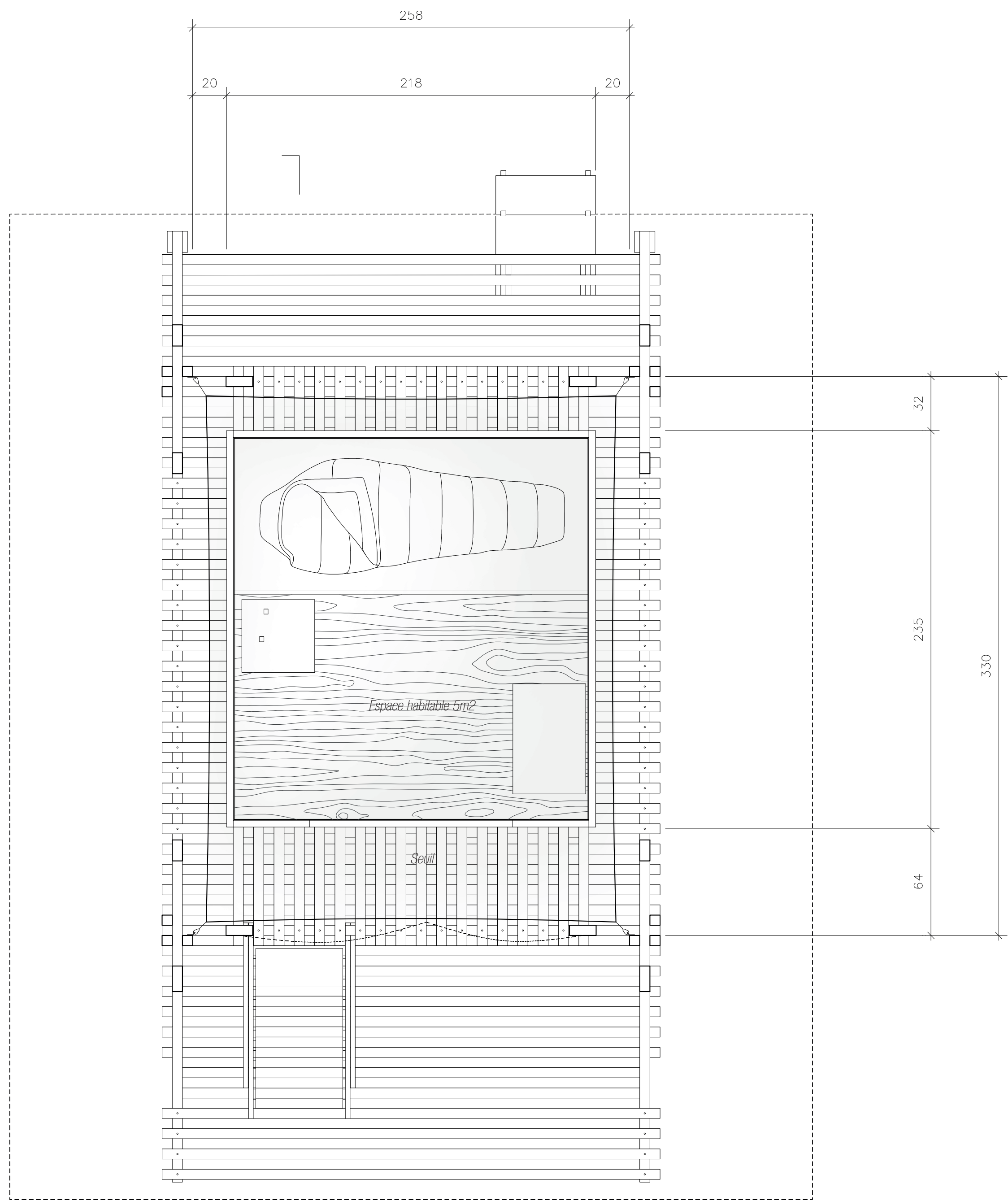
Plan niveau supérieur 1.20
