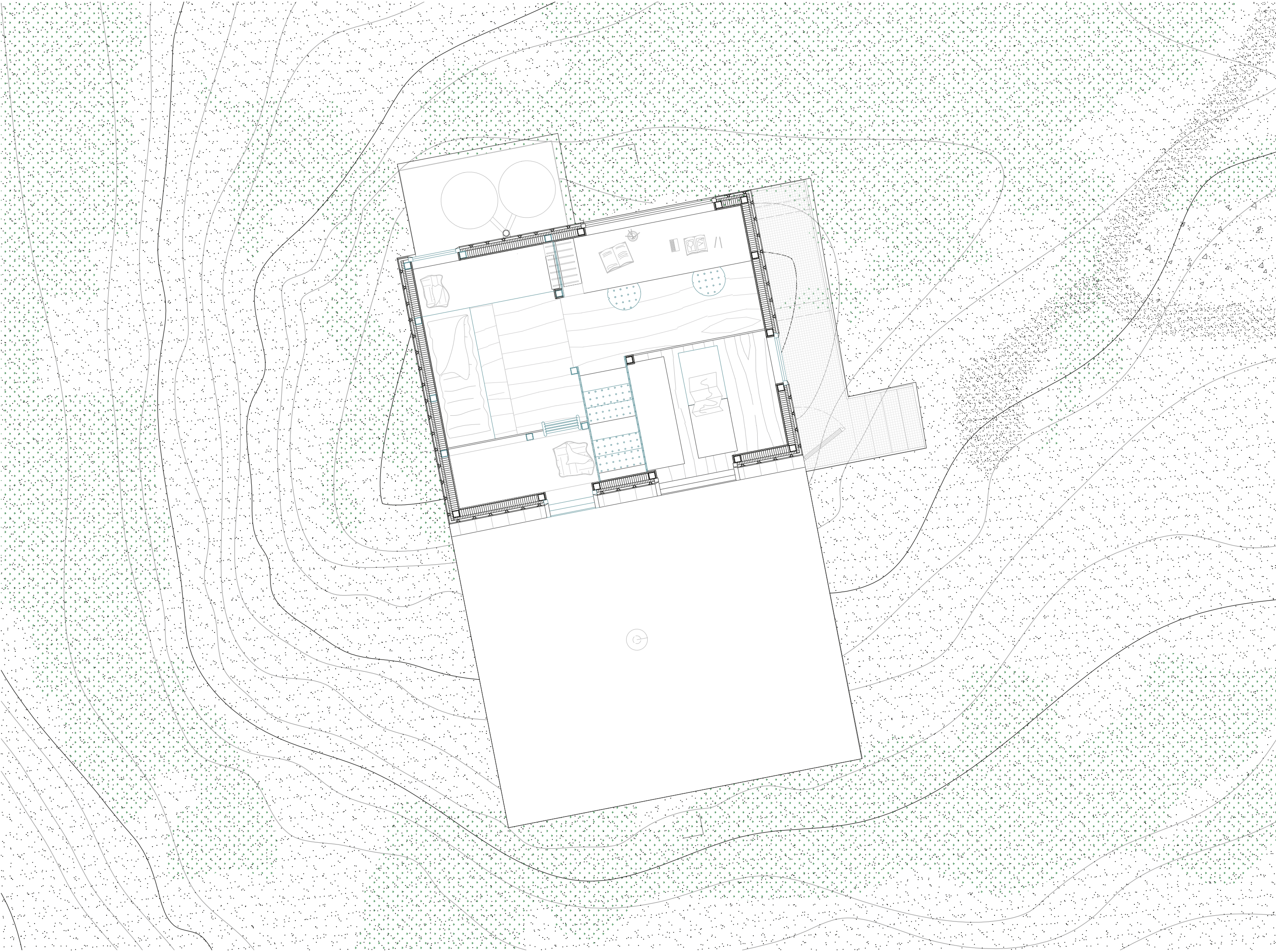
Plan étage 1:50
