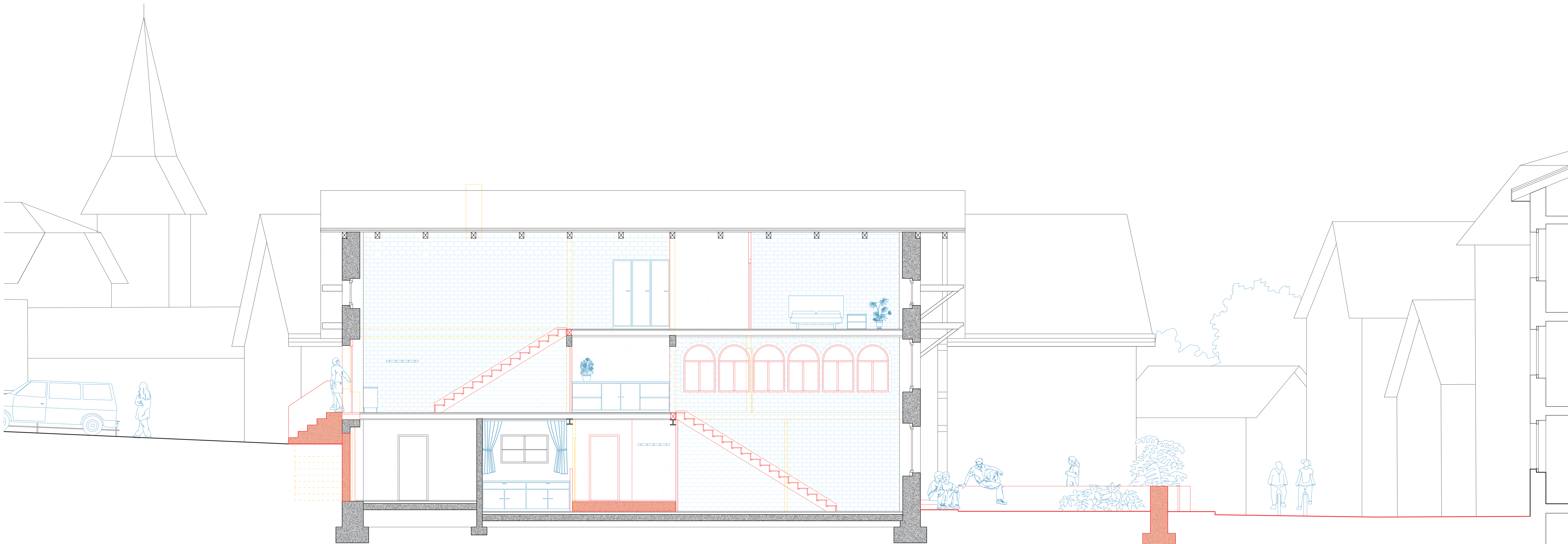
COUPE LONGITUDINALE CC' / 1:50
