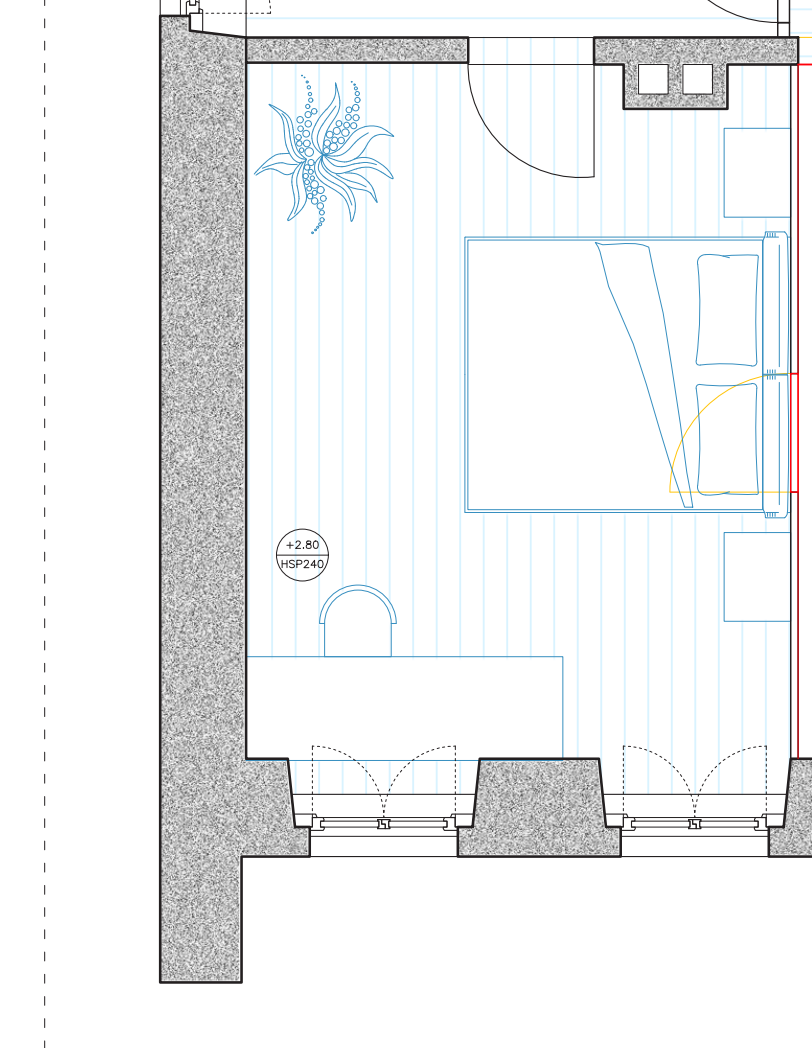
PLAN 1ER ÉTAGE / 1:50
