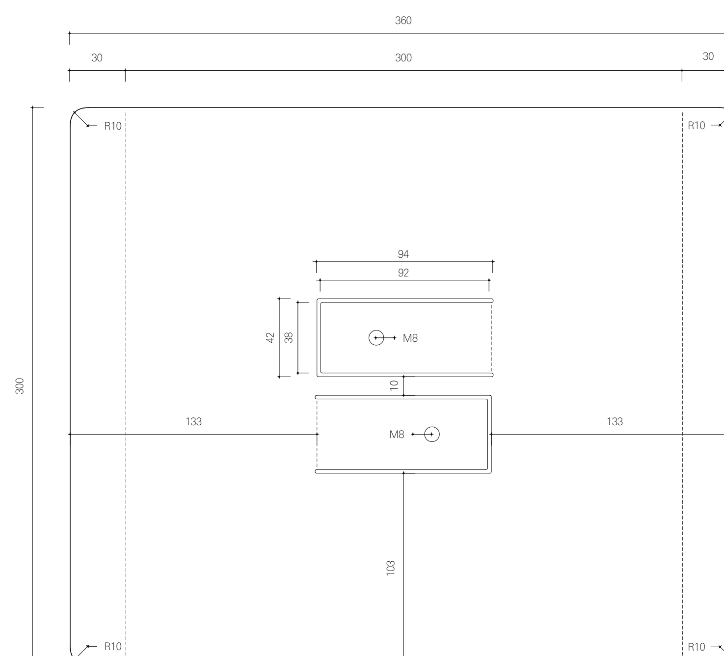
Déplié Tôle Tablette
