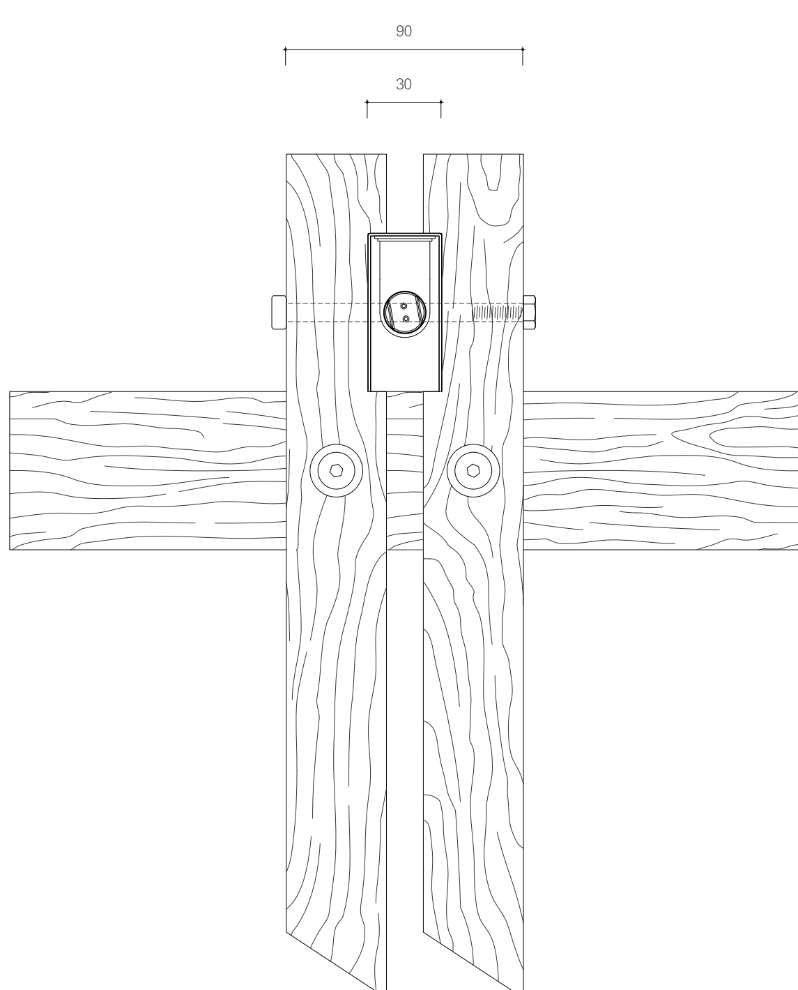
Coupe Luminaire
