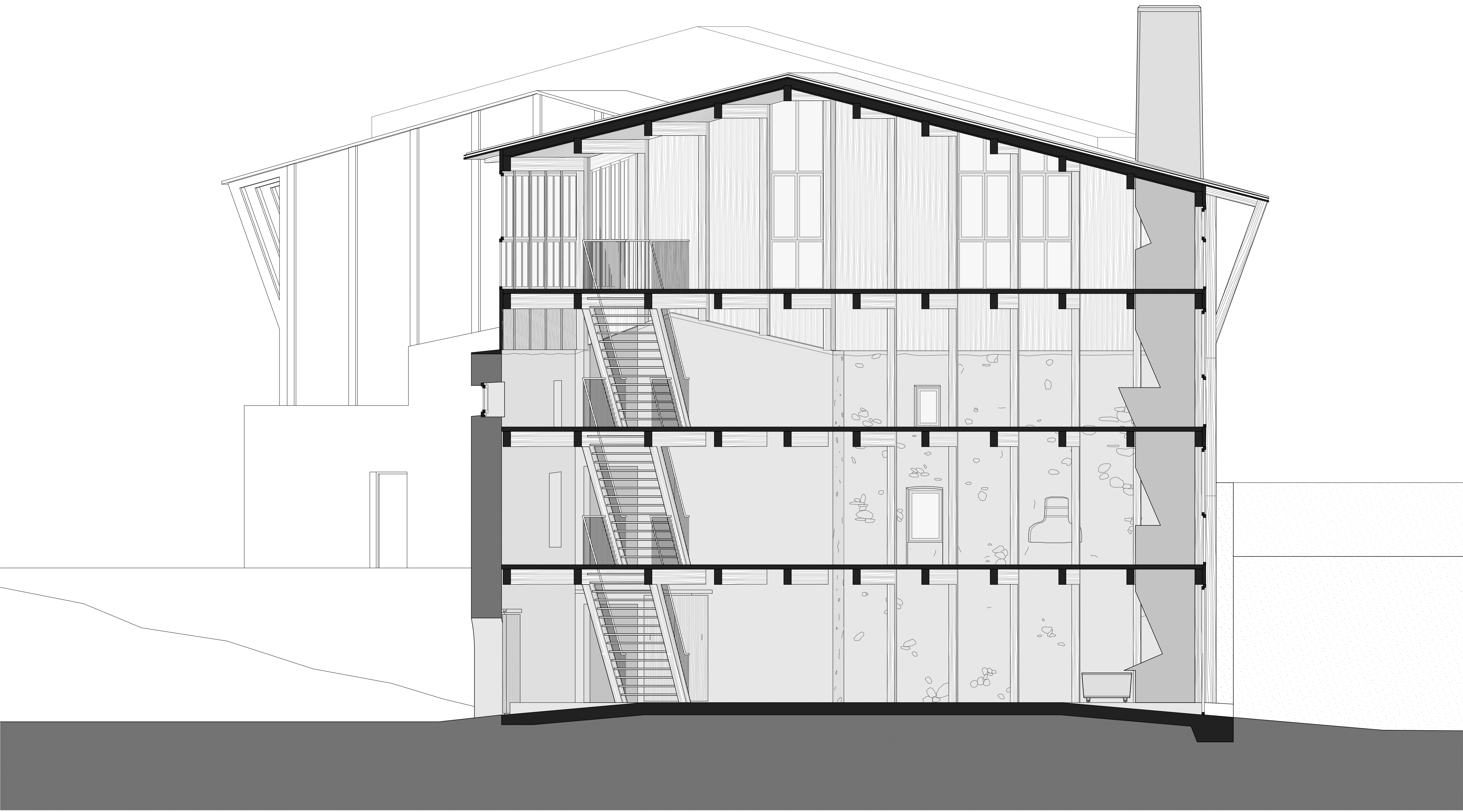
ELEVATION DD | 1:50
