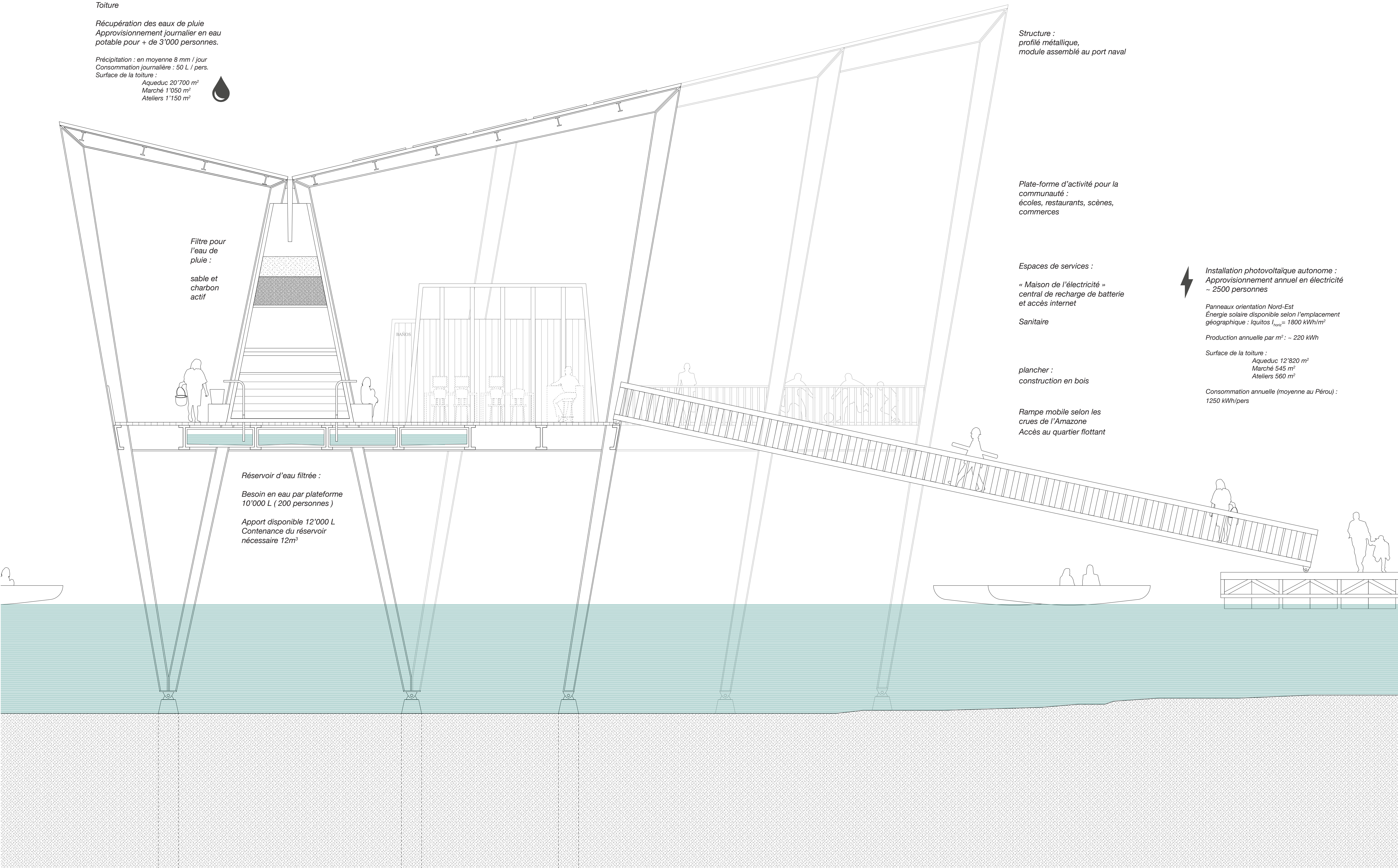
Coupe constructive 1:50
