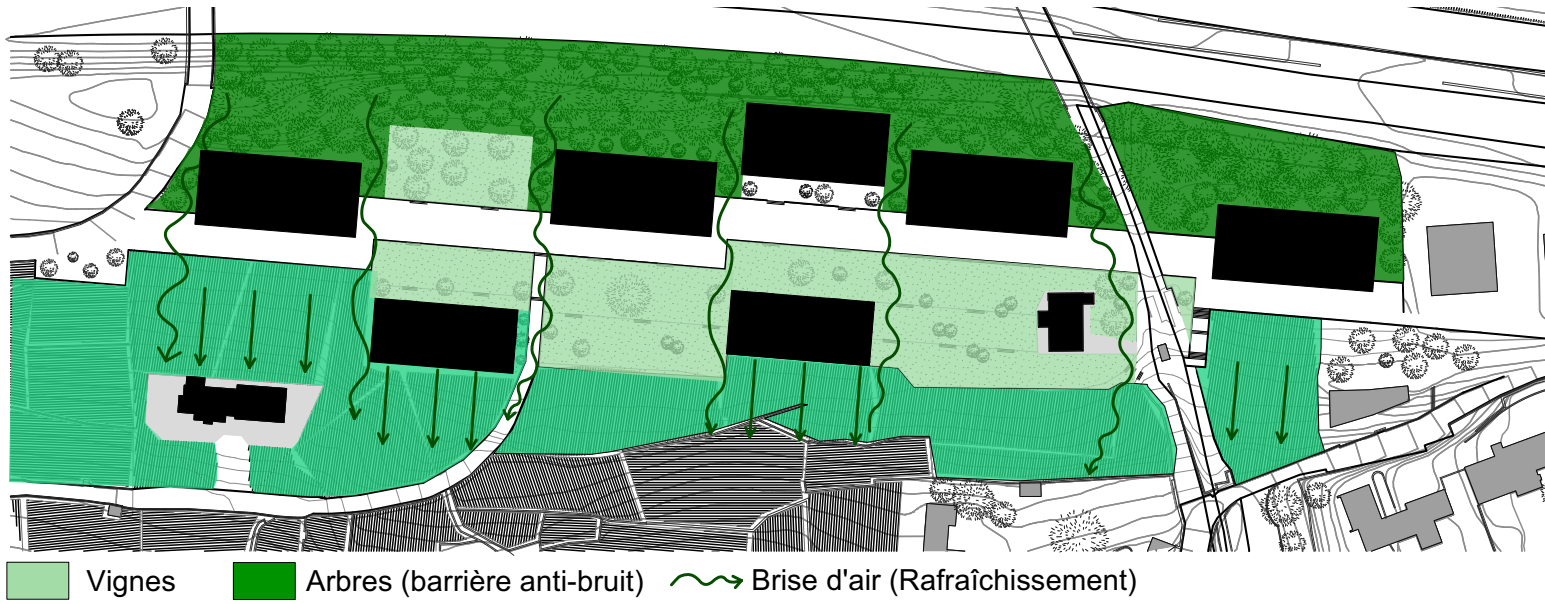
Schéma bioclimatique
