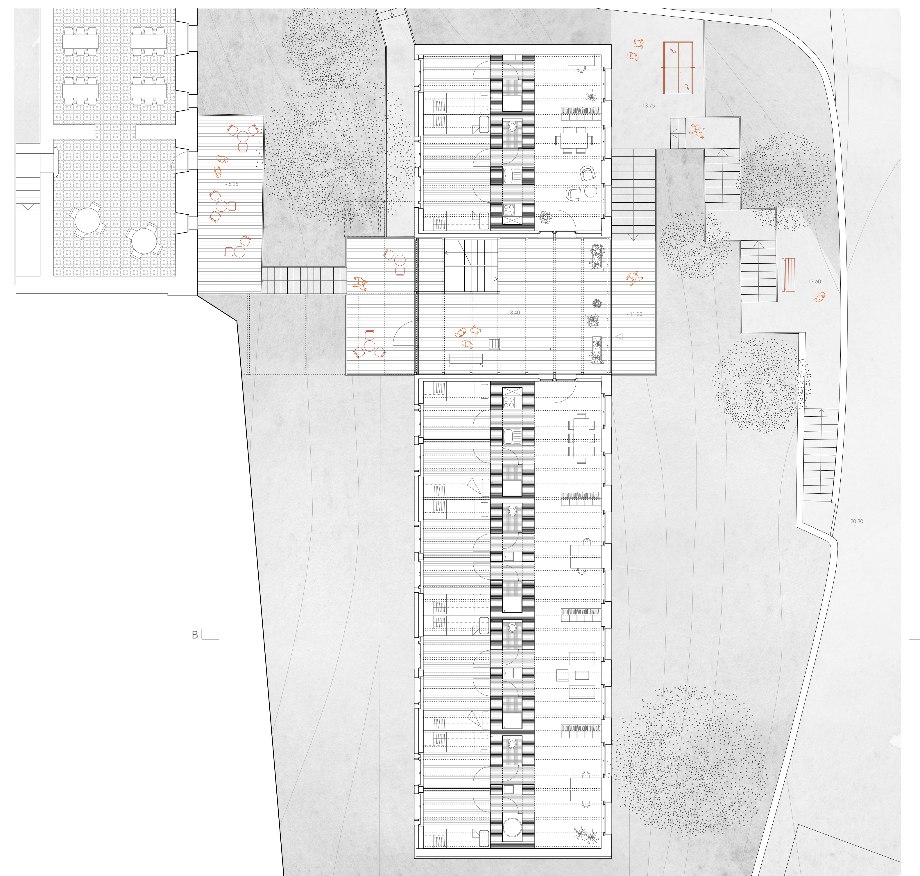
Plan accès niveau inférieur 1:100
