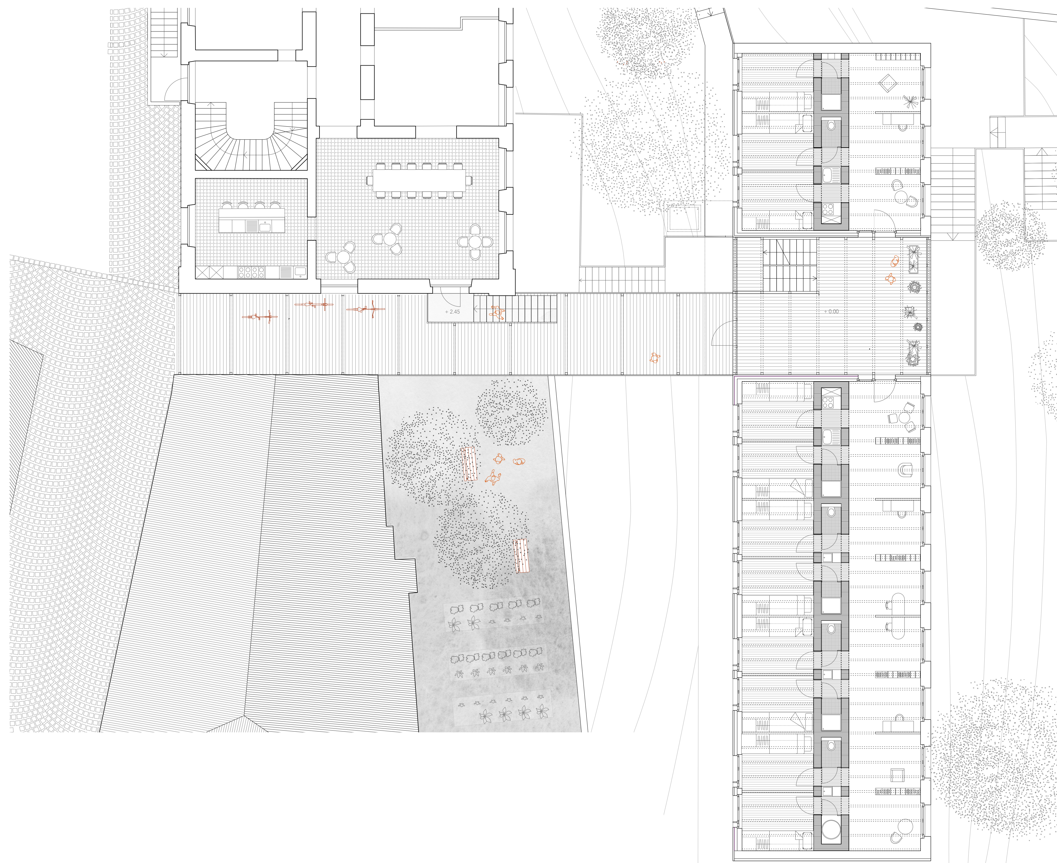
Plan accès Cité 1:100
