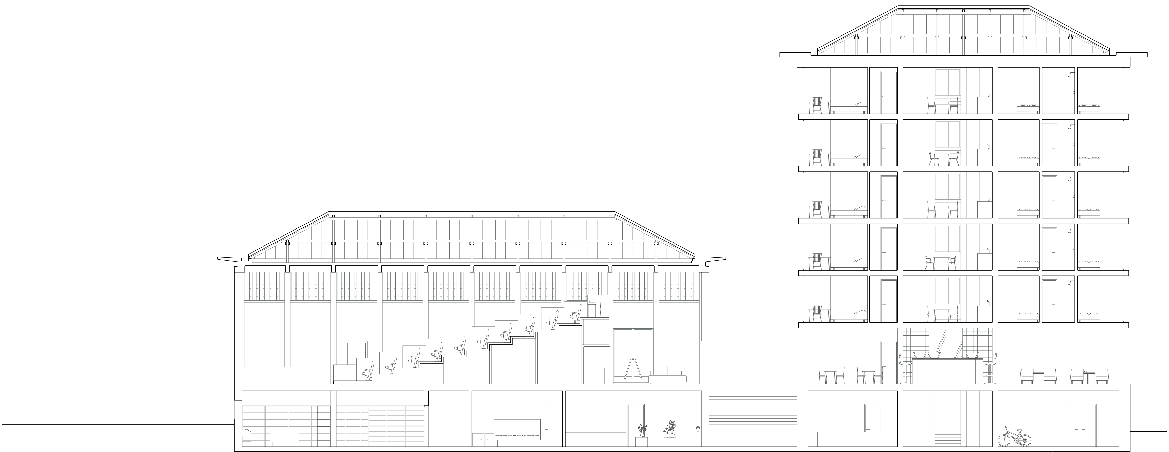
Coupe 1:100
