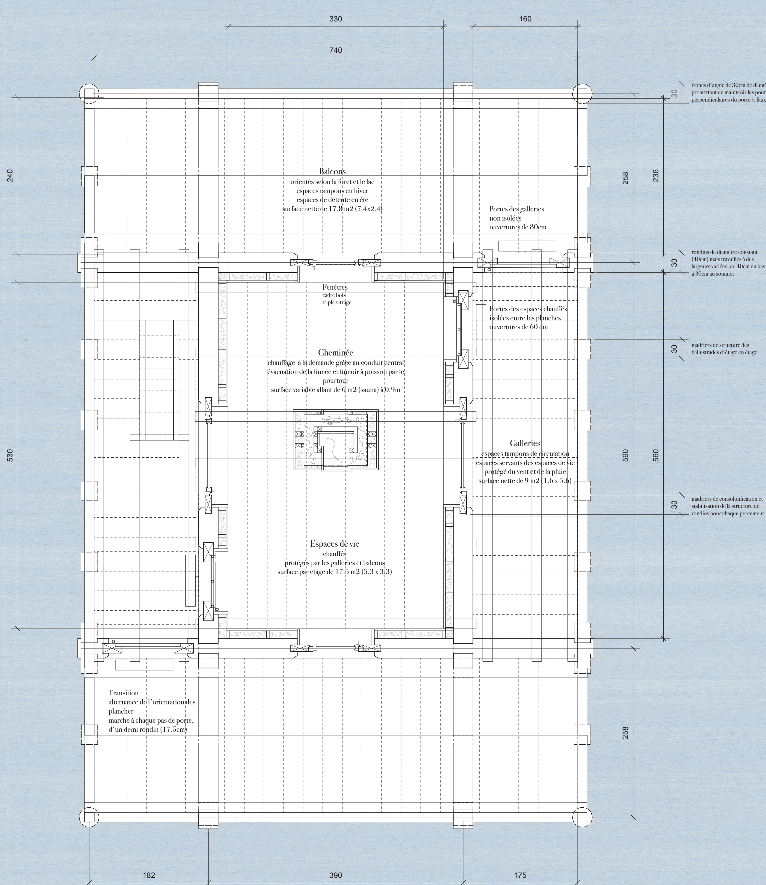
Plan étage I 1:33
