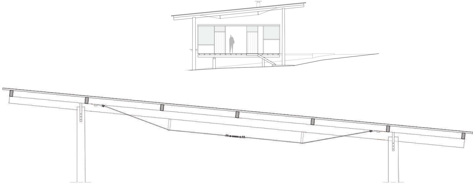
AMPLIAÇÃO SEÇÃO TIPO VC01 1:25
